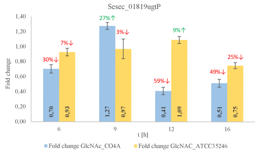
Graf 27: Změna relativní míry exprese genu u kmene CO4A a ATCC35246
