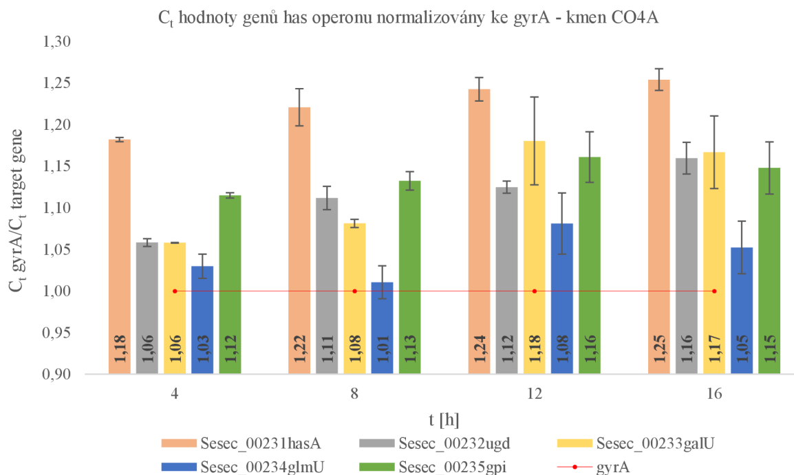
Graf 6: Normalizované C_t hodnoty genů has operonu kmene CO4A. has operon je regulován dvěma konzervovanými promotory. Míra exprese odpovídá předpokladu. Gen kódující hasA měl nejvyšší expresi ze všech sledovaných genů. Míra exprese genů klesá se vzdáleností od promotorové oblasti, tak jak ukazují data v grafu. Výjimku tvoří gen Sesec_00235 (gpi), který kóduje enzym klíčový pro dráhy energetického metabolismu. Je tedy pravděpodobná možnost samostatné regulace a proto je před genem umístěna druhá promotorová sekvence regulující expresi pouze gpi genu [31].
