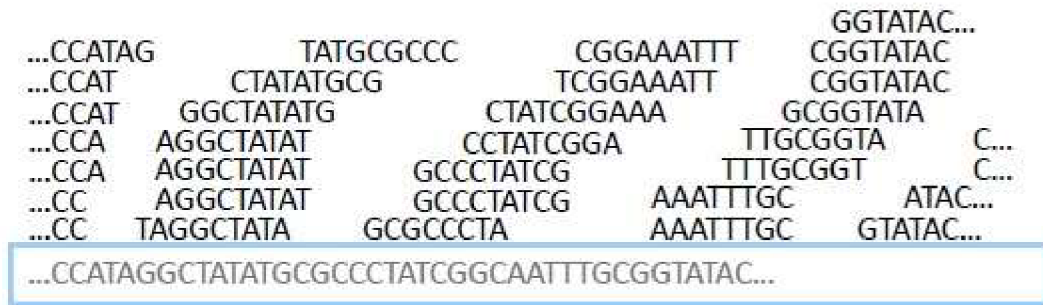
Obrázek 9: Sestavování delších sekvencí DNA (contigů) z krátkých úseků, které byly získány sekvenací. Modrým rámečkem je vyznačená sekvence contigu získaného z překrývajících se sekvencí [62].
