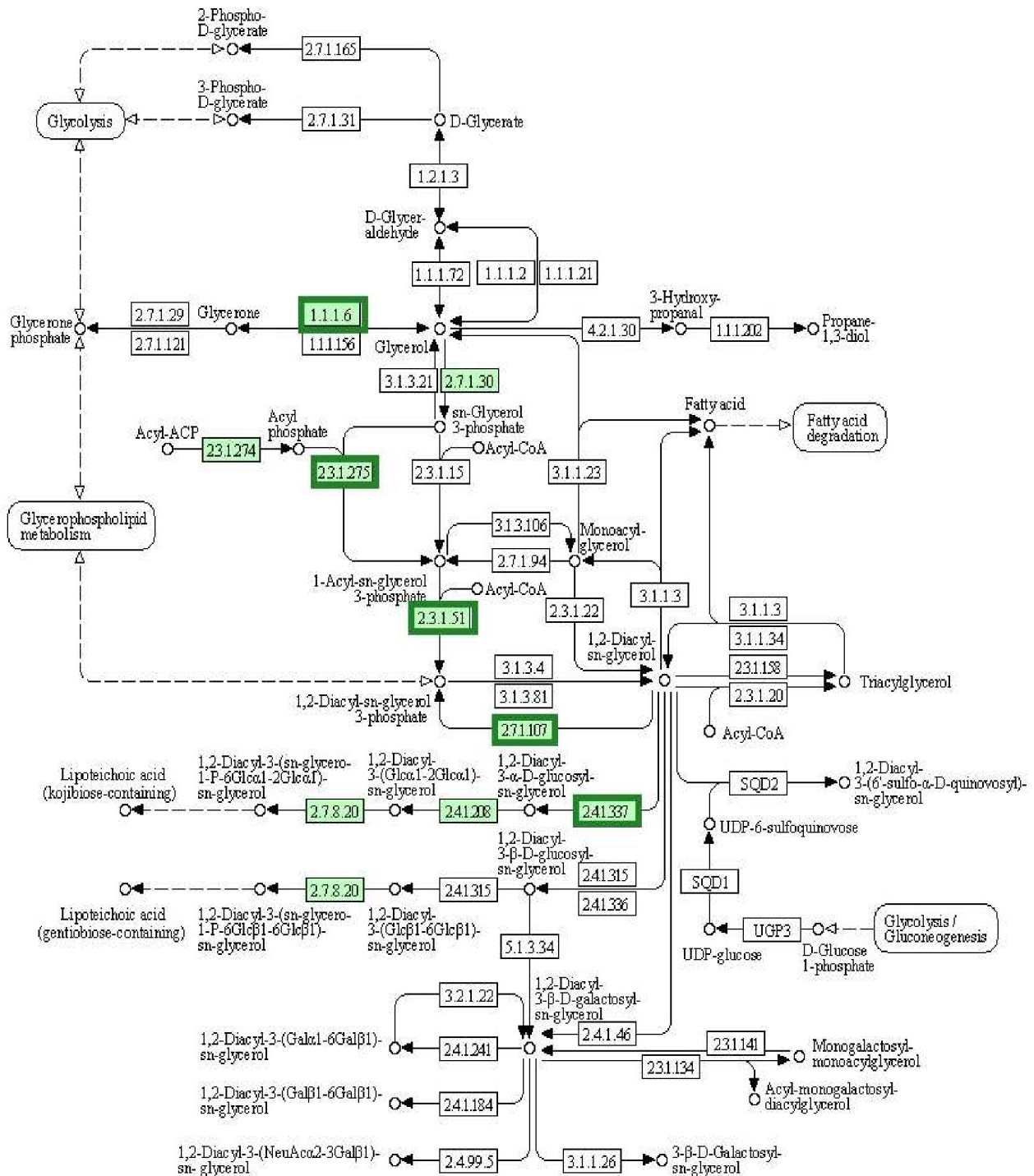
Obrázek 14: Metabolické dráhy glycerolipidů jsou spojeny s energetickým metabolismem především přes dráhy glykolýzy. Byly sledovány geny centrálních drah transformace glycerolu. Výstupem těchto drah jsou například triacylglyceroly a další cukerné alkoholy, ale také kyselina lipoteichoová. Kyselina teichoová je součástí buněčné stěny, ale ne v takové míře jako předcházející peptidoglykan. Dráha není výrazně kompetitivní s dráhou syntézy HA. Mohla by ovlivňovat energetický metabolismus prostřednictvím drah degradace lipidů (nebylo testováno). Vyznačeny jsou geny (zeleně orámováni) se změnou exprese vyšší než 10 %. Zeleně podbarvené geny se vyskytují u S. zooepidemicus ATCC35246. Bíle podbarvené geny nejsou u S. zooepidemicus přítomny. [upraveno dle 130]
