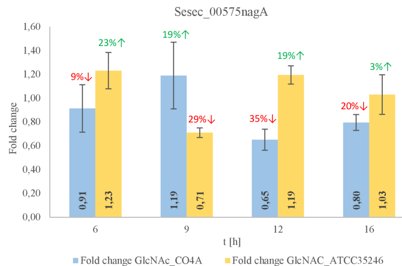
Graf 16: Změna relativní míry exprese genu u kmene CO4A a ATCC35246
