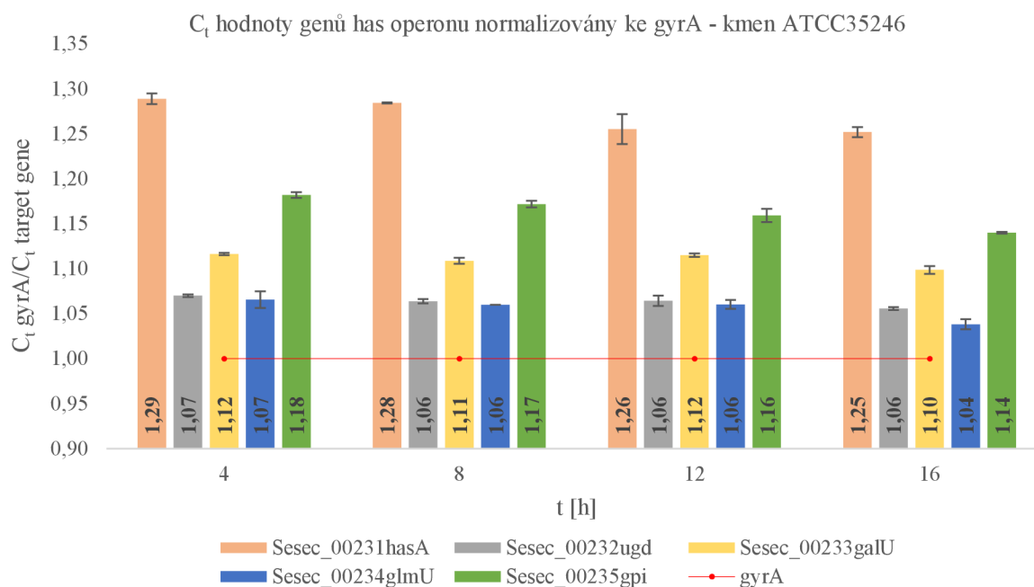
Graf 7: U kmene ATCC35246 byl vývoj exprese genů stejný jako u kmene CO4A. Dokonce u ATCC35246 byla relativní míra exprese hasA ve 4. hodině kultivace vyšší než u CO4A. Ostatní geny měly míru exprese srovnatelnou s CO4A.
