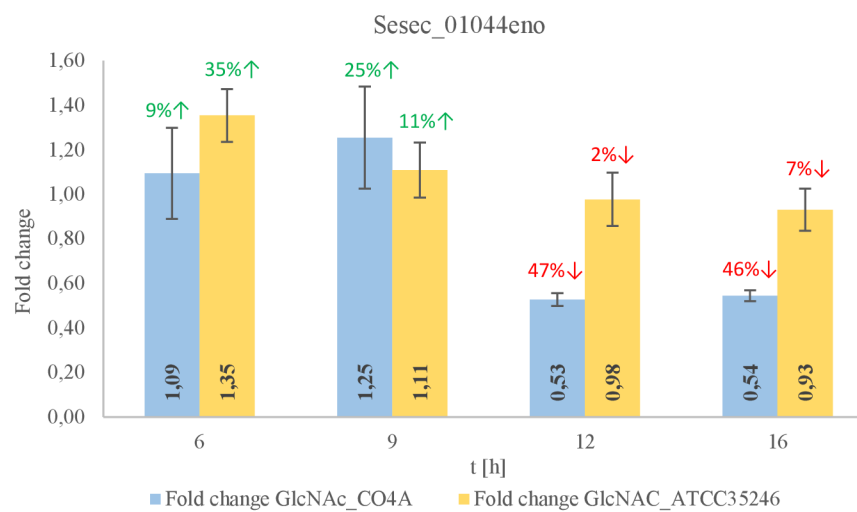
Graf 19: Změna relativní míry exprese genu u kmene CO4A a ATCC35246
