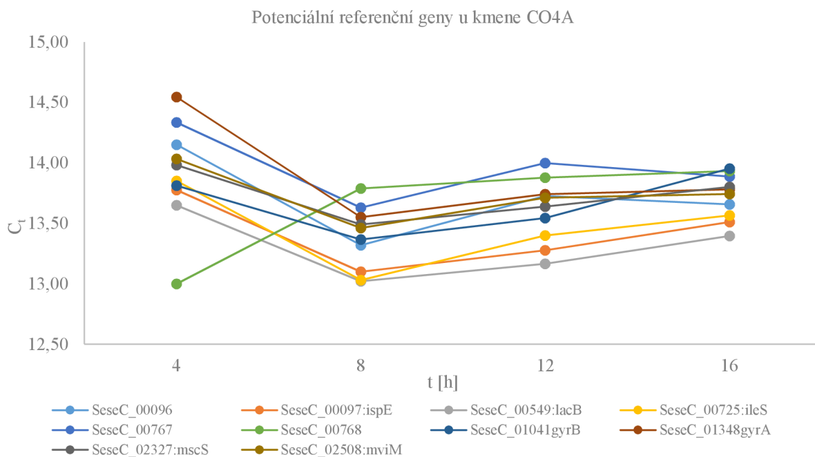
Graf 2: V grafu jsou uvedeny výsledné hodnoty C_t , pro první biologický replikát kmene CO4A. Z grafu jsou patrné průběhy exprese vybraných genů. Z těchto dat byl hodnocen průběh křivky genu ve srovnání s ostatními potenciálními referenčními geny.
