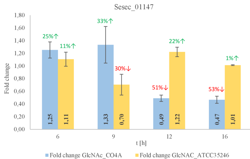
Graf 20: Změna relativní míry exprese genu u kmene CO4A a ATCC35246
