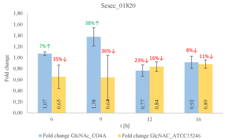
Graf 28: Změna relativní míry exprese genu u kmene CO4A a ATCC35246
