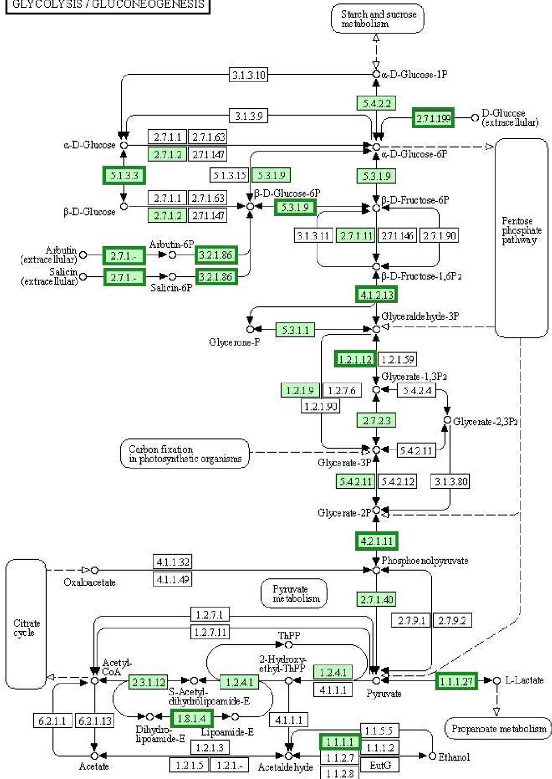
Obrázek 10: Na obrázku jsou vyznačeny zeleným orámováním sledované geny metabolických drah části energetického metabolismu S. zooeconomicus se změnou míry exprese vyšší než 10 % (poměr exprese genu v kmeni CO4A vůči kmeni ATCC35246). Zeleně podbarvené geny se vyskytují u S. zooeconomicus . Bíle podbarvené geny nejsou u S. zooeconomicus přítomny. [upraveno dle 130]
