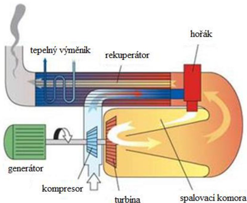
Obr. 13 Mikroturbína [31]
