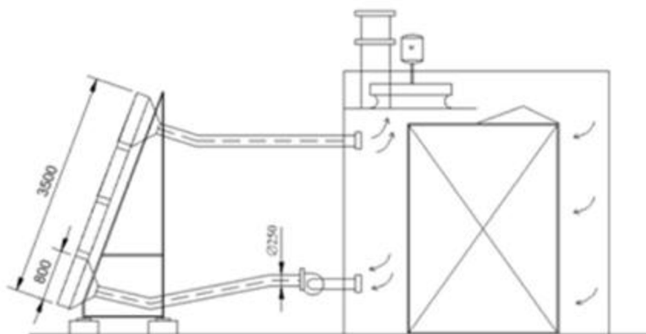
Obr. 17 Schéma komorové sušárny řeziva se slunečním kolektorem [35]
