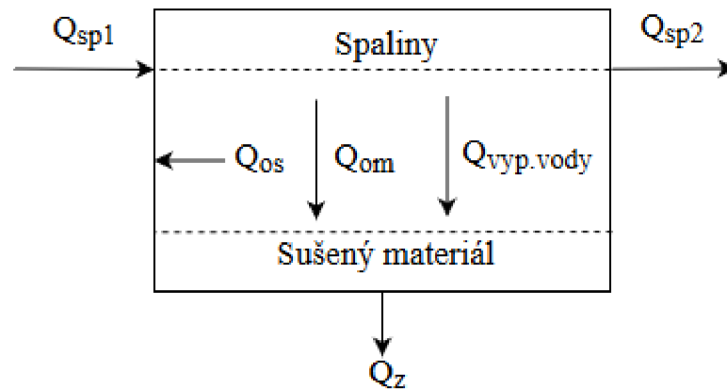
Obr. 24 Schéma bubnové sušárny
