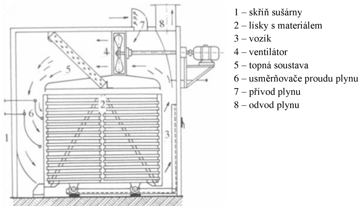
Obr. 3 Komerová sušárna [12]
