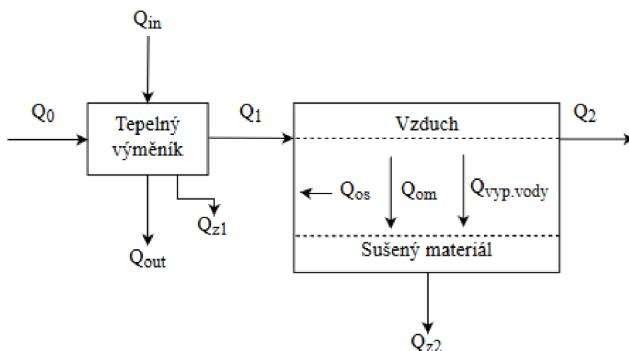
Obr. 21 Schéma komorové sušárny s otevřeným oběhem
