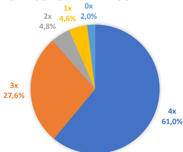
Graf 2 – Usnášeníschopnost hlasování
