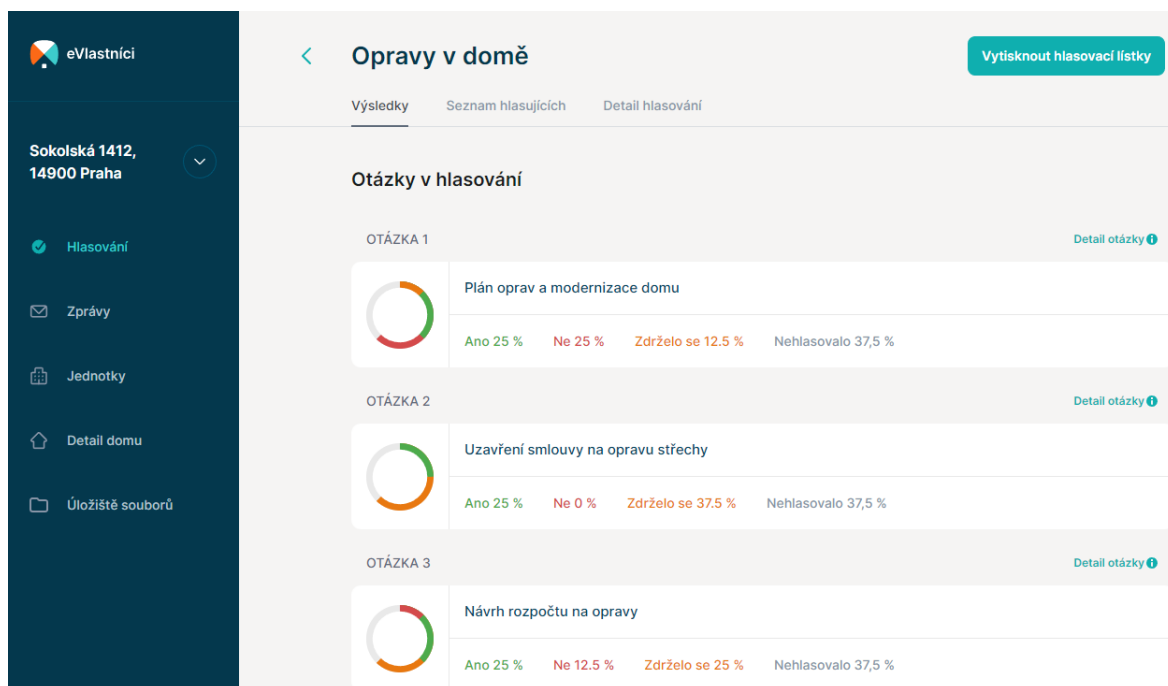
Obrázek 15 – Detail hlasování
