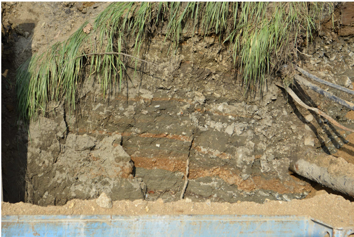
Obr. 13 Vrstvy svahu
