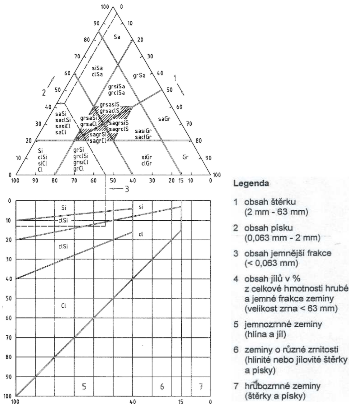
Obr. 30 Diagram pro zatřídění zemin ( http://geotech.fce.vutbr.cz/text.html )
