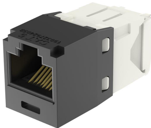
Obrázok 13: Mini-Com® Cat 6 UTP RJ45 TG Jack Module Panduit (15)
