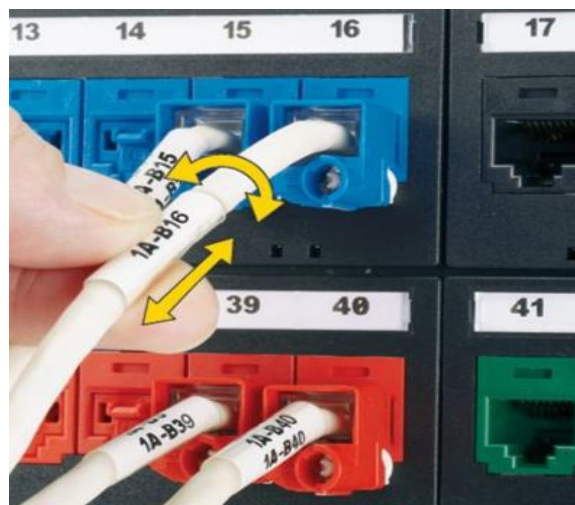
Obrázok 21: Štítok na značenie kabeľáže Panduit (23)
