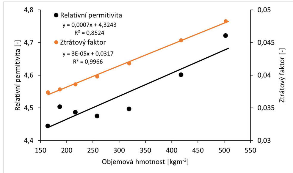
Obr. 17: Závislost relativní permitivity a ztrátového faktoru na objemové hmotnosti při 1 MHz u vzorku S15
