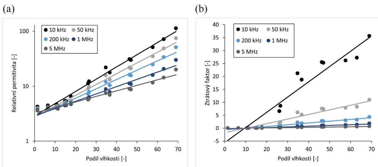
Obr. 11: Závislosti mezi podílem vlhkosti, relativní permitivitou a ztrátovým faktorem u vybraných frekvencích u smrku při výšce materiálu 15,7 mm. (a) - závislost relativní permitivity na podílu vlhkosti, (b) - závislost ztrátového faktoru na podílu vlhkosti
