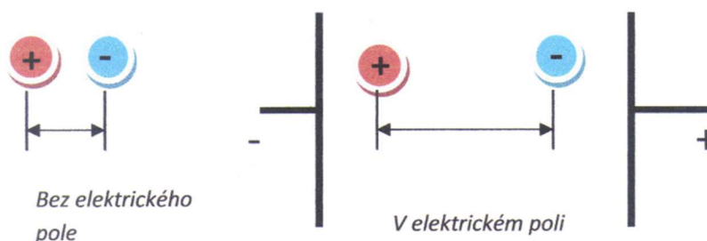
Obr. 6: Iontová polarizace [5]
