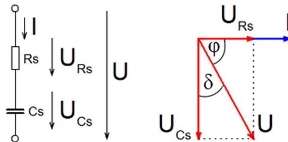
Obr. 3: Sériové zapojení s fázorovým diagramem [14]
