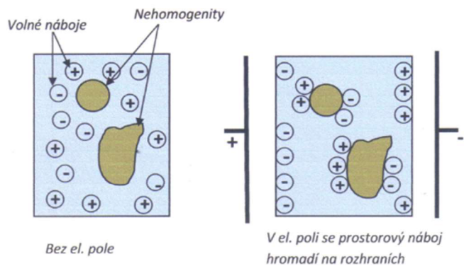
Obr. 8: Migrační polarizace [5]
