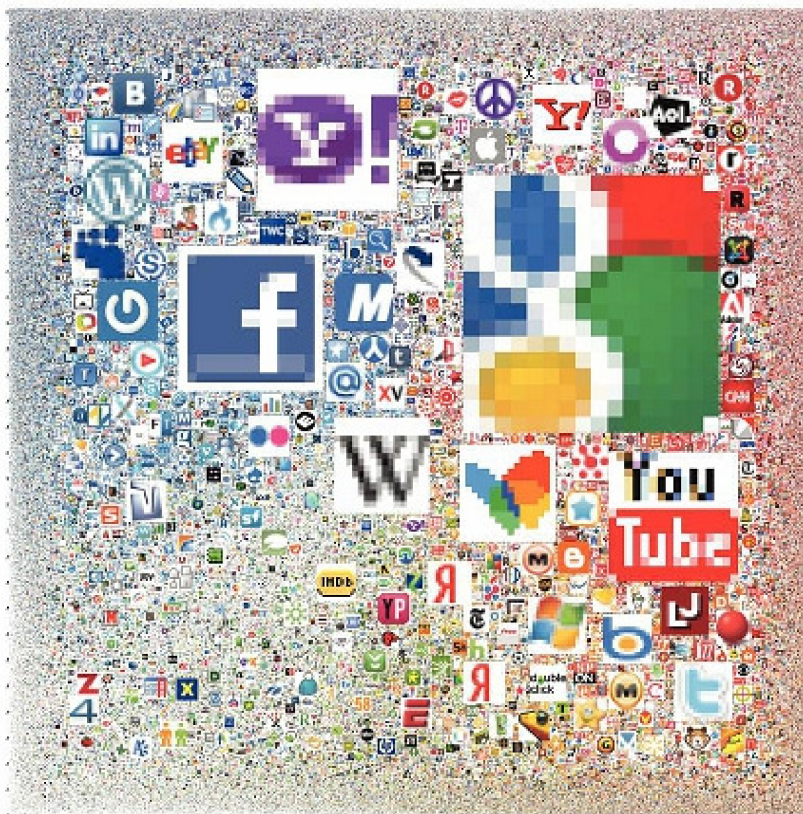
Obr. 3: Ikony webu (18)
