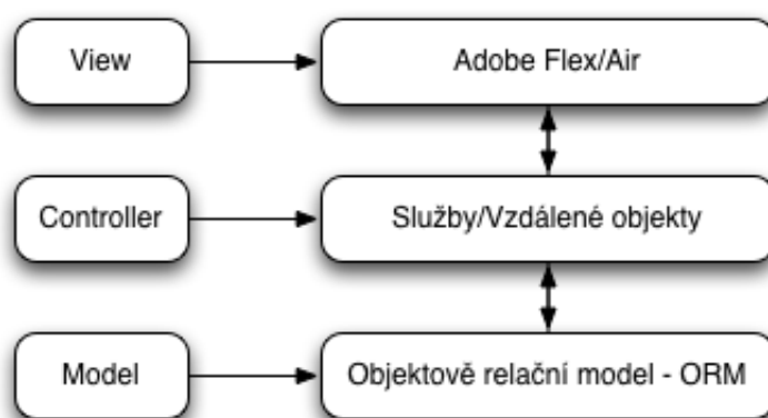
Obrázek 4.1: Vrstvový model
