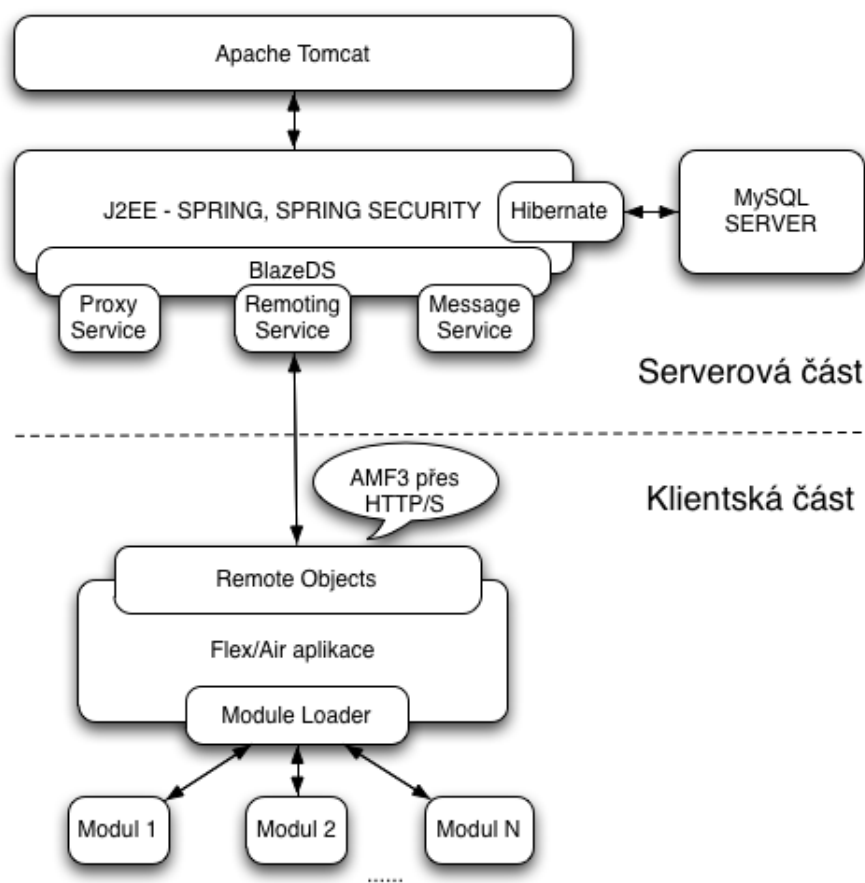
Obrázek 3.2: Struktura aplikace
