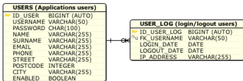
Obrázek 4.2: Relace 1:N
