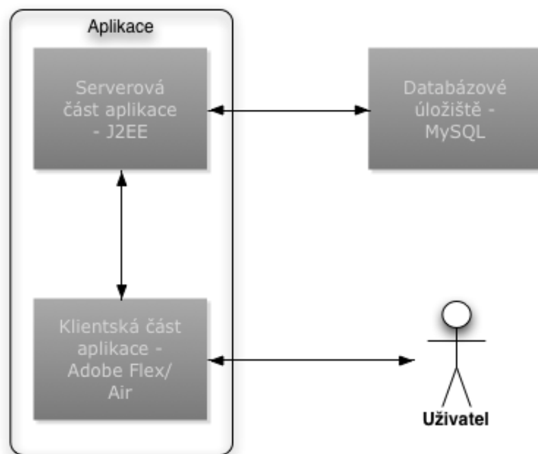
Obrázek 3.1: Komunikační struktura
