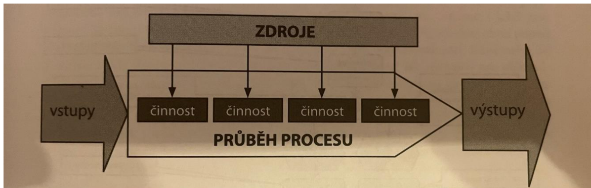
Obrázek 7- Schéma procesu.
