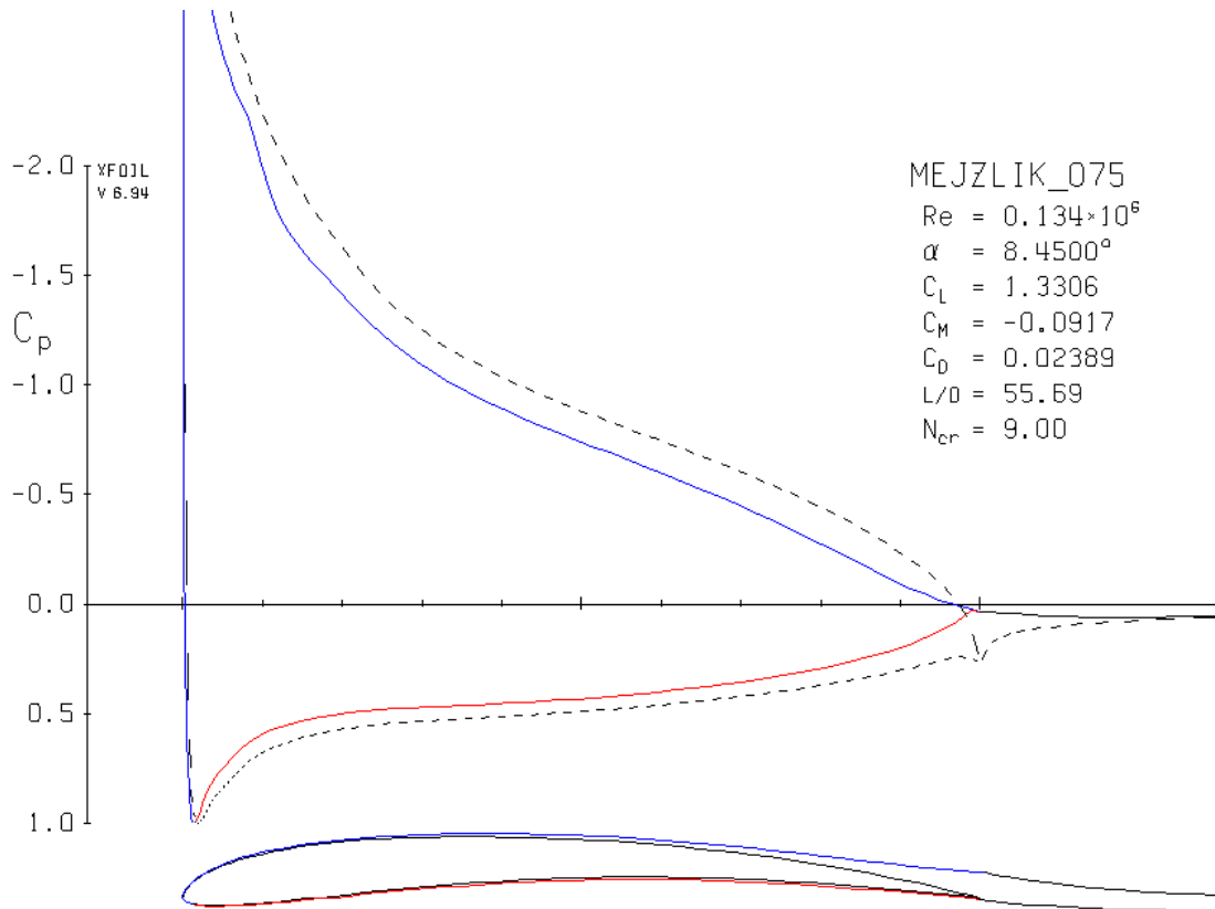
Obrázek 2.7: Příklad výpočtu rozložení tlaku v XFOilu.
