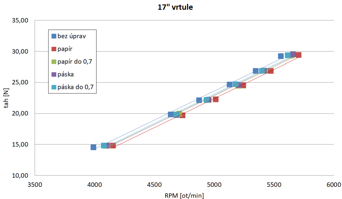
Obrázek 3.17: Porovnání účinností 17" vrtule s úpravami nosných ploch.
