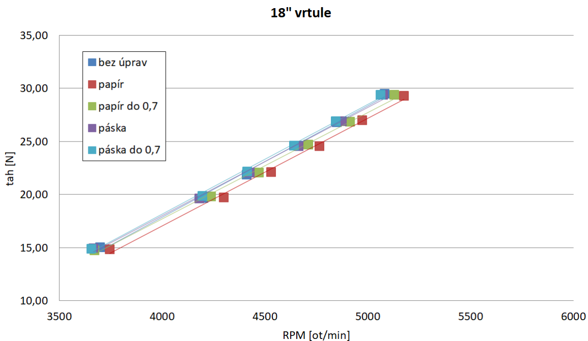
Obrázek 3.18: Porovnání účinností 18" vrtule s úpravami nosných ploch.
