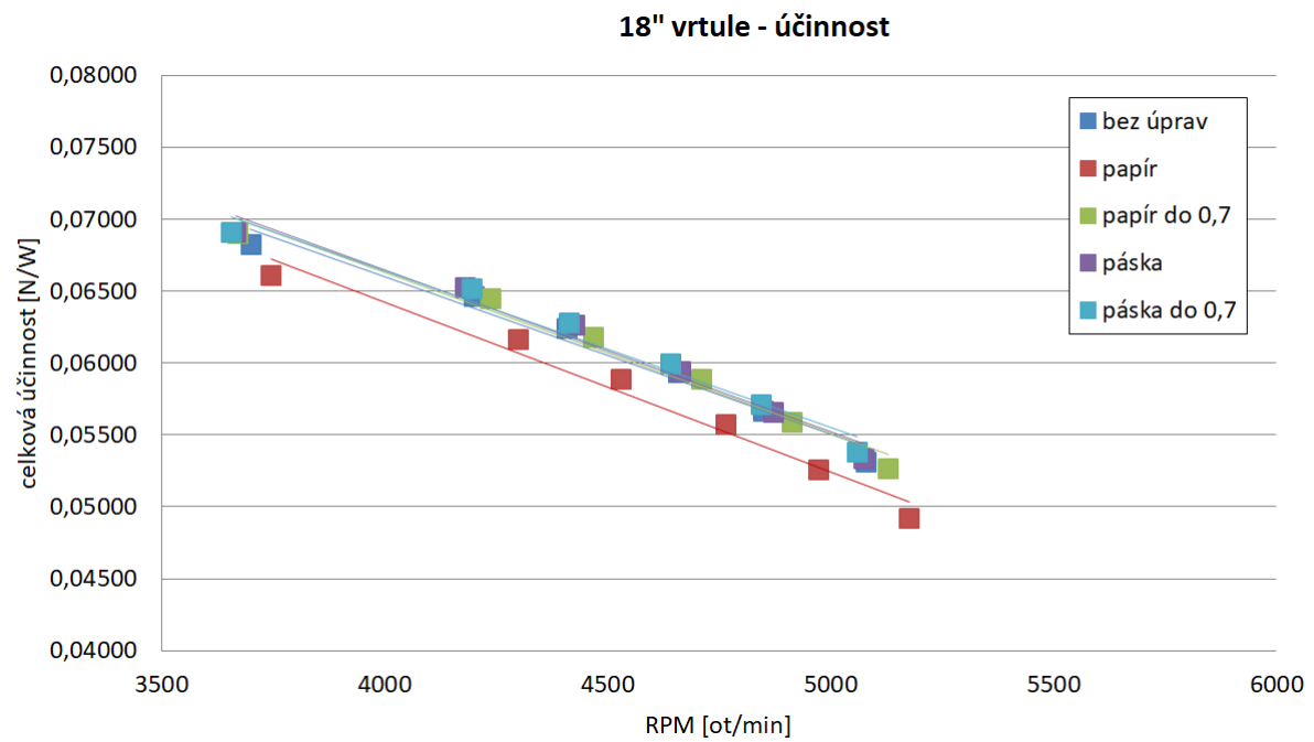
Obrázek 3.20: Srovnání účinnosti 18" vrtule s různými úpravami.
