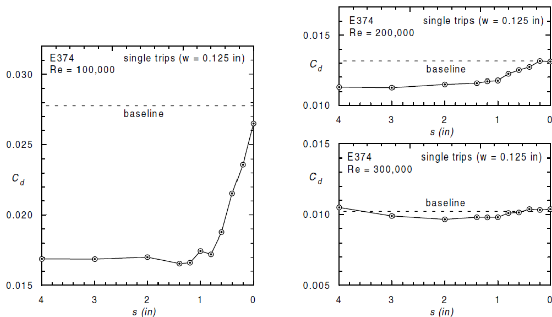
Obrázek 1.28: Závislost koeficientu odporu na pozici turbulátorové pásky pro Reynoldsova čísla 1 \cdot 10^5 , 2 \cdot 10^5 a 3 \cdot 10^5 . s = 0 odpovídá pozici 46 % délky tělivy a s = 4 odpovídá 13 % délky tělivy. [28]
