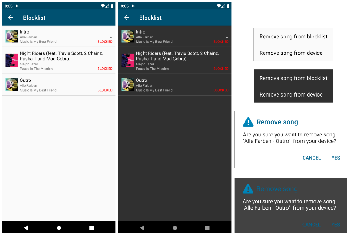
Obr. 6.15: Obrázok vľavo a v strede zobrazuje obrazovku so zoznamom blokovaných pesničiek. Prvé dva obrázky vpravo hore zobrazujú vyskakovacie menu, ktoré sa zobrazí po dlhom kliknutí na položku tohto zoznamu. Na spodných dvoch obrázkoch vpravo je dialógové okno, ktoré sa zobrazí, keď užívateľ zvolí akciu pre vymazanie pesničky zo zariadenia z vyskakovacieho menu a cez ktoré musí užívateľ svoju voľbu potvrdiť, ak chce pesničku zo zariadenia skutočne vymazať.
