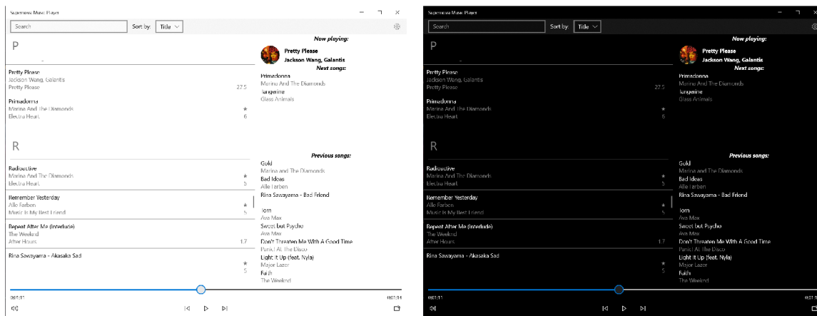
Obr. 6.18: Obrázky zobrazujú celú hlavnú obrazovku počítačovej verzie hudobného prehrávača vo svetlom a v tmavom režime. Hlavná obrazovka pozostáva zhora nadol zo systémového titulného panelu, titulného panelu aplikácie, panelu s pesničkami a z ovládacieho panelu. Všetky tieto časti sú detailnejšie zobrazené na ďalších obrázkoch.
