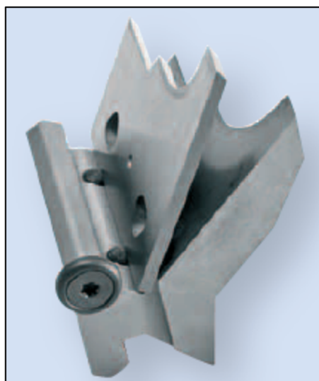
Obr. 32 Nožový segment s VBD [3].
