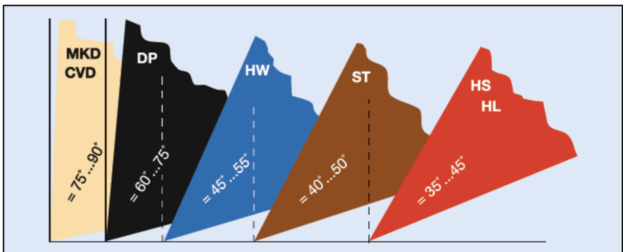
Obr. 4 Úhel břitu v závislosti na nástrojovém materiálu [3].
