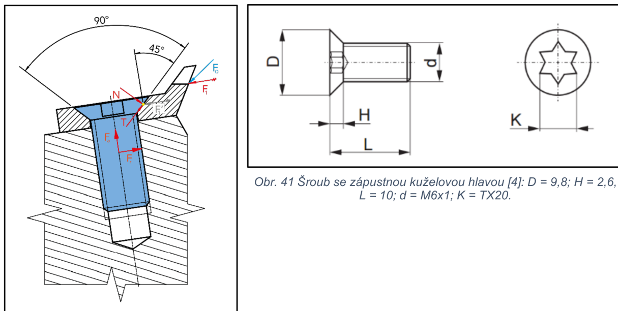
Obr. 40 Rozložení řezného odporu na upínací šroub: F_0 – řezný odpor, F_1 – složka řezného odporu působící v tečném směru, F_a – axiální síla ve šroubu, F_r – radiální síla ve šroubu, N , T – reakční síly hlavy šroubu.
