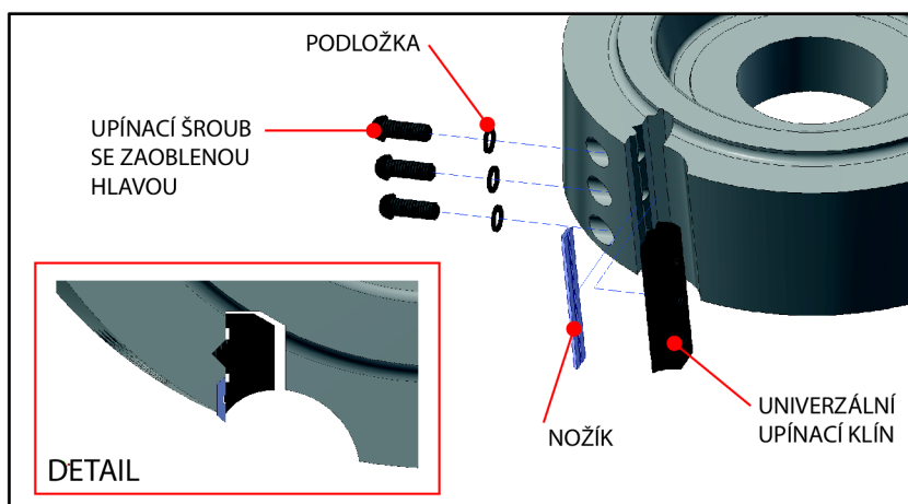
Obr. 23 Upínací systém univerzálních nožů firmy Vydon [5].
