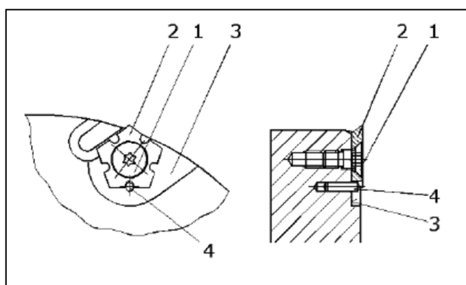
Obr. 24 Zajištění polohy čepem (4) [6].
