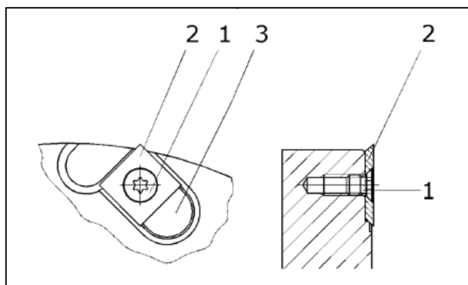
Obr. 25 Zajištění polohy tvarováním lůžka VBD [6].
