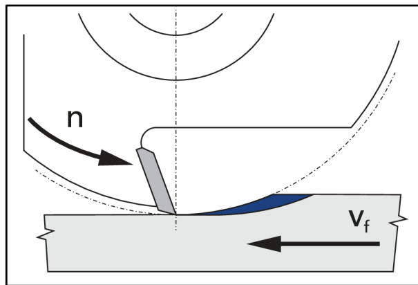
Obr. 8 Nesousledné frézování [4].
