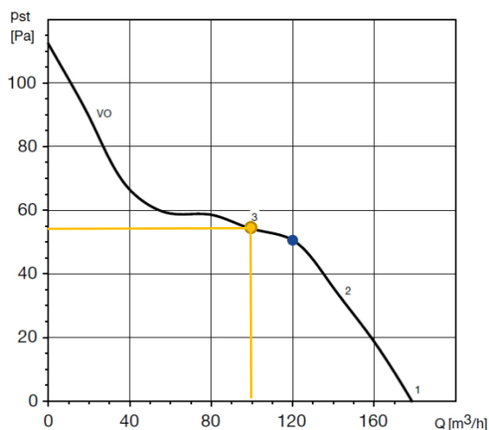
Graf 11 Stanovení statického tlaku V9
