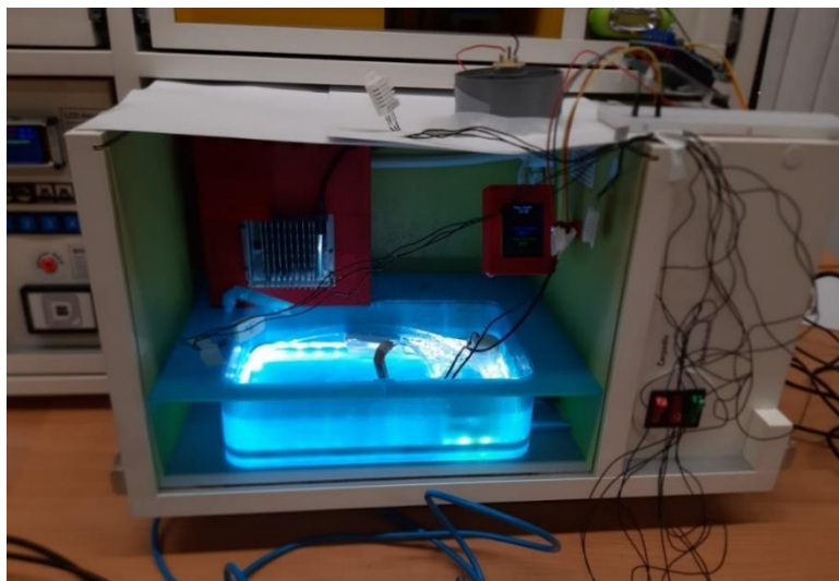
Obr. 55 Model bazénové haly
