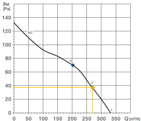
Graf 3 Stanovení statického tlaku V1
