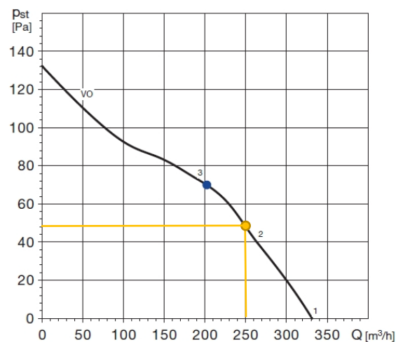
Graf 6 Stanovení statického tlaku V4
