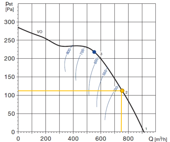
Graf 5 Stanovení statického tlaku V3
