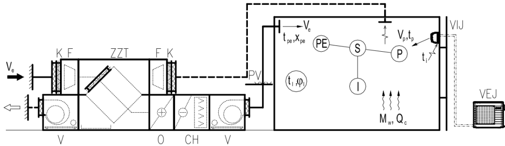
Obr. 46 Schéma provozu [23]
