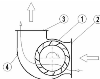
Obr. 11 Diametrální ventilátor (1 - oběžné kolo, 2 - sání, 3 - výtlak, 4 - skříň) [21]
