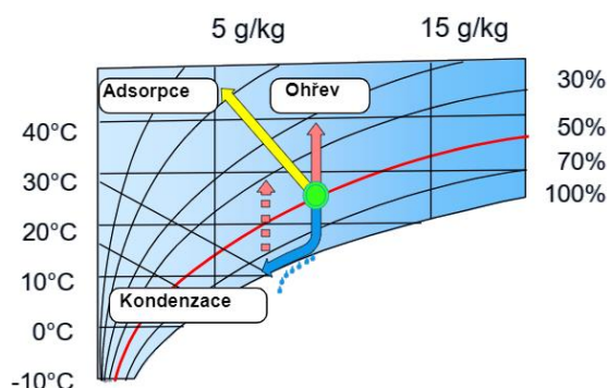
Obr. 15 Metody odvlhčování [33]
