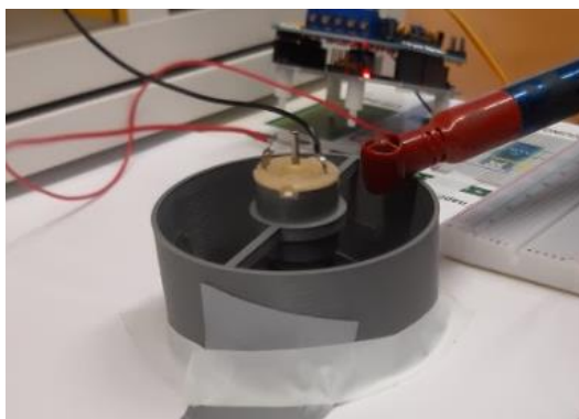
Obr. 57 Vrtulový a žahavý anemometr
