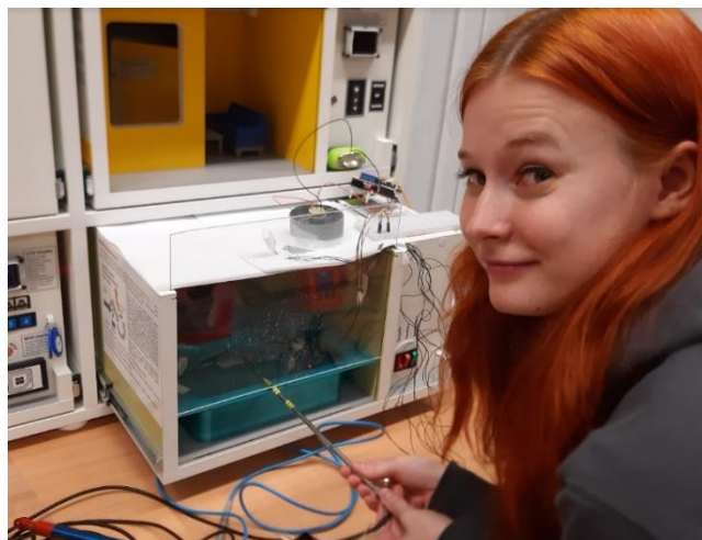
Obr. 61 Měření rychlosti vzduchu nad hladinou
