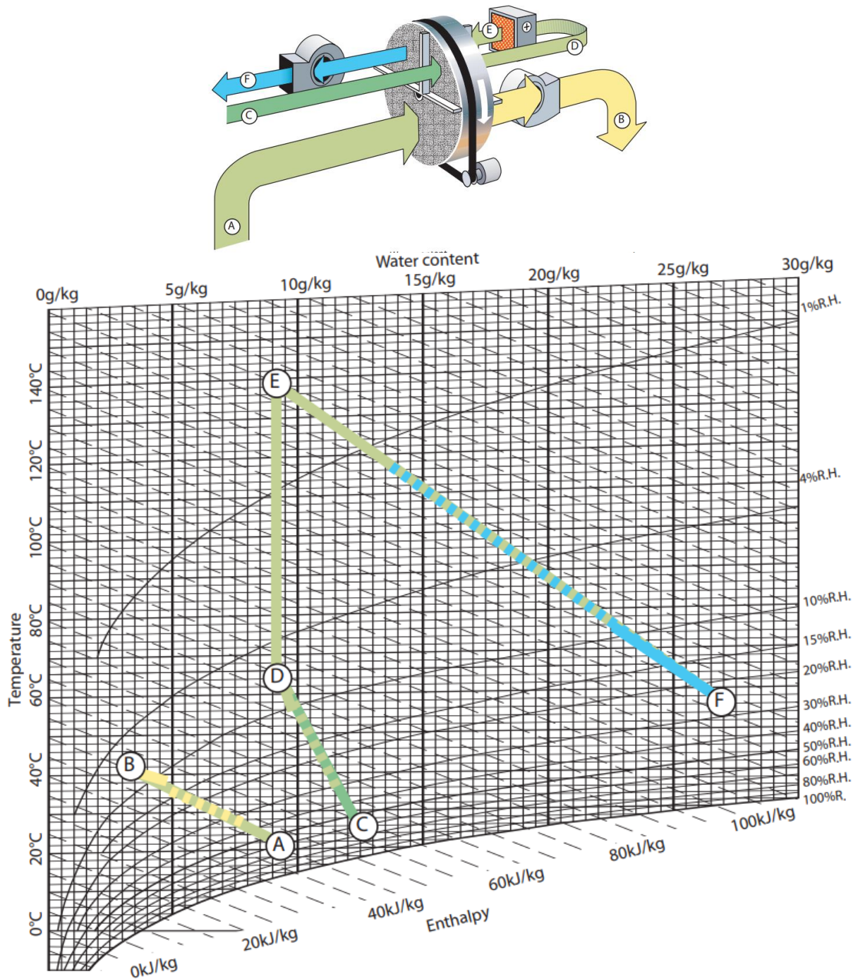
Obr. 54 Proces odvlhčení v HX – diagramu [33]
