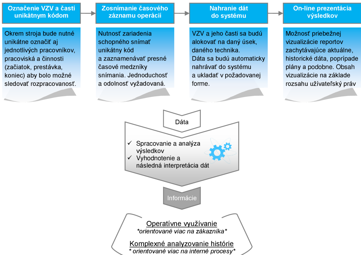
Obrázok 4.2 Všeobecný proces navrhovaného monitoringu repasíí.
