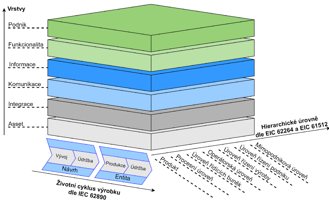
Obr. 2.1: Referenční architektonický model pro průmysl 4.0.
