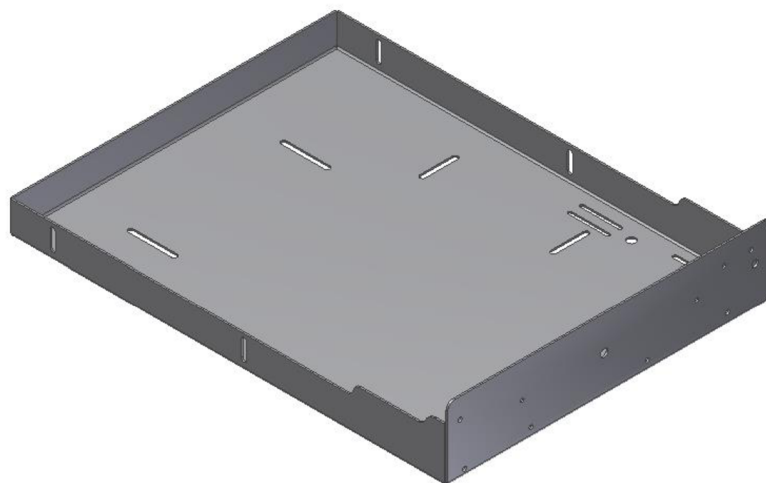
Obr. 4.7.5 3D model zásobníka.
