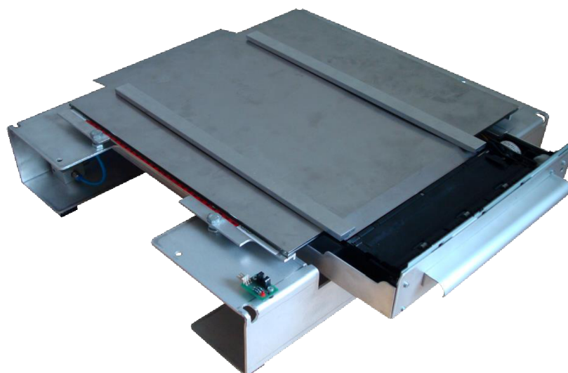
Obr. 4.7.2 Hliníková zostava základacieho mechanizmu.
