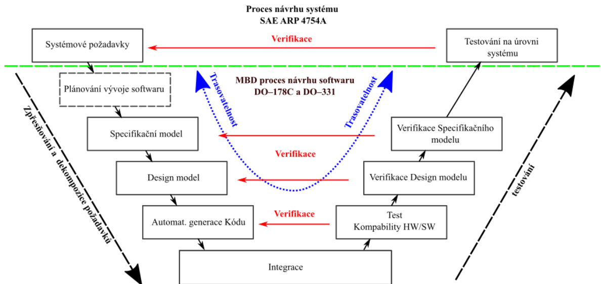
Obrázek 2: Příklad V-modelu podle DO-178C a DO-331
