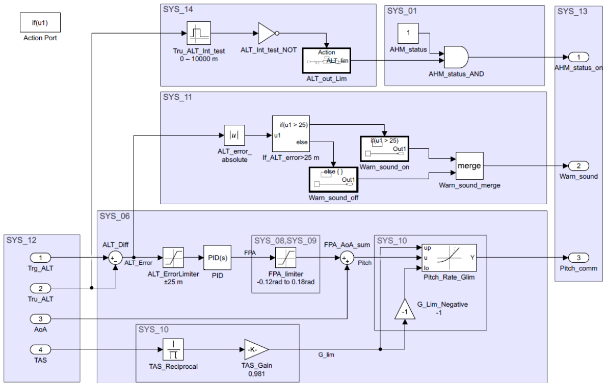
Obrázek 6: Kontrolní logika AHM autopilota
