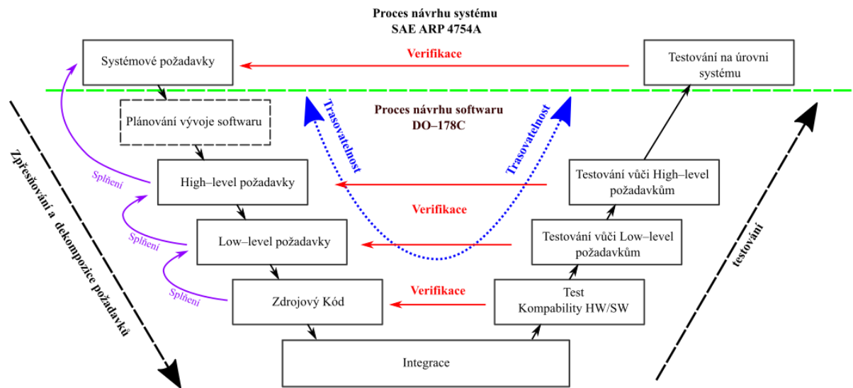
Obrázek 1: V-model pro DO-178C
