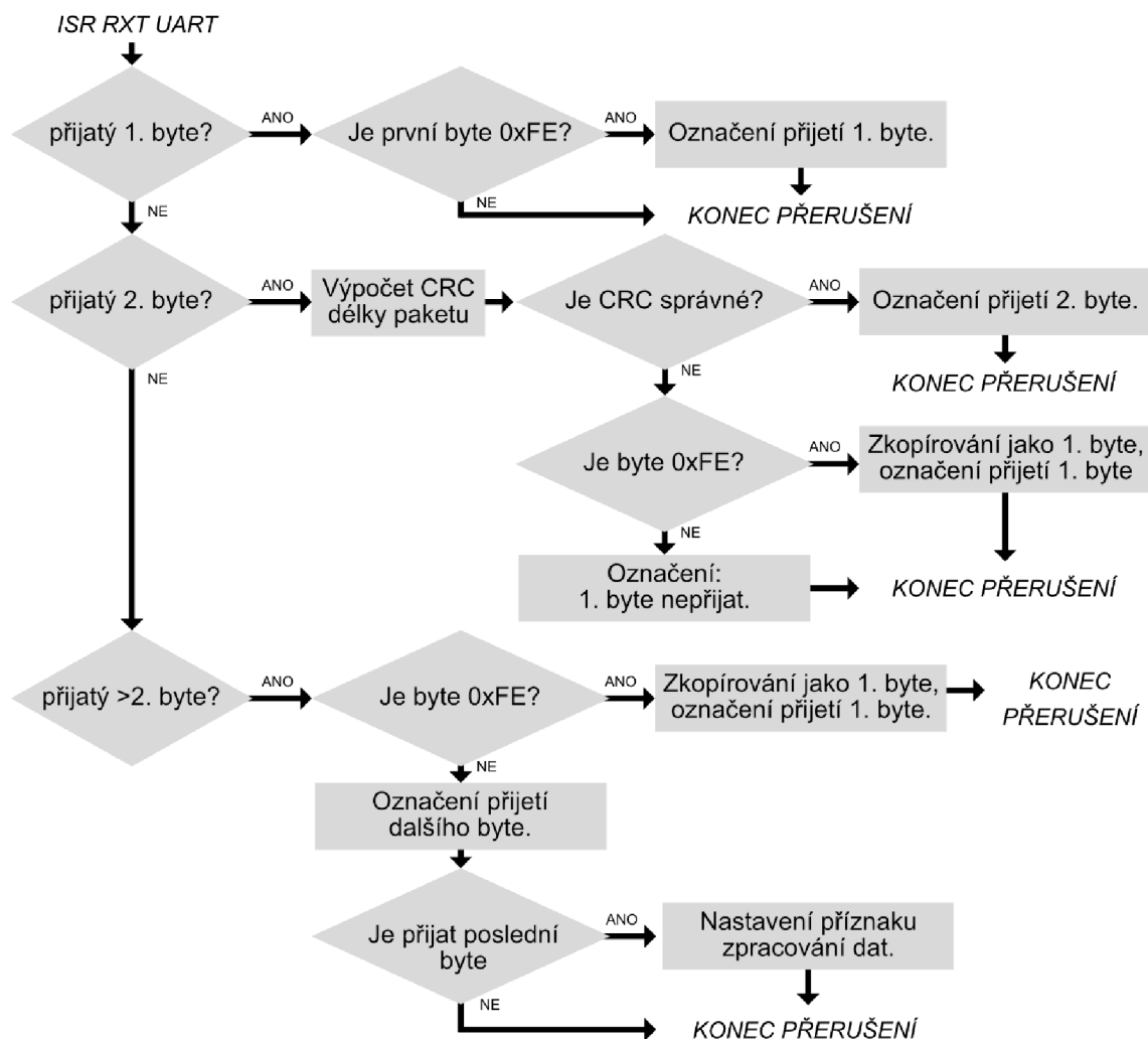
Obrázek 6.1 Vývojový diagram obsluhy přerušeni RXT UART
