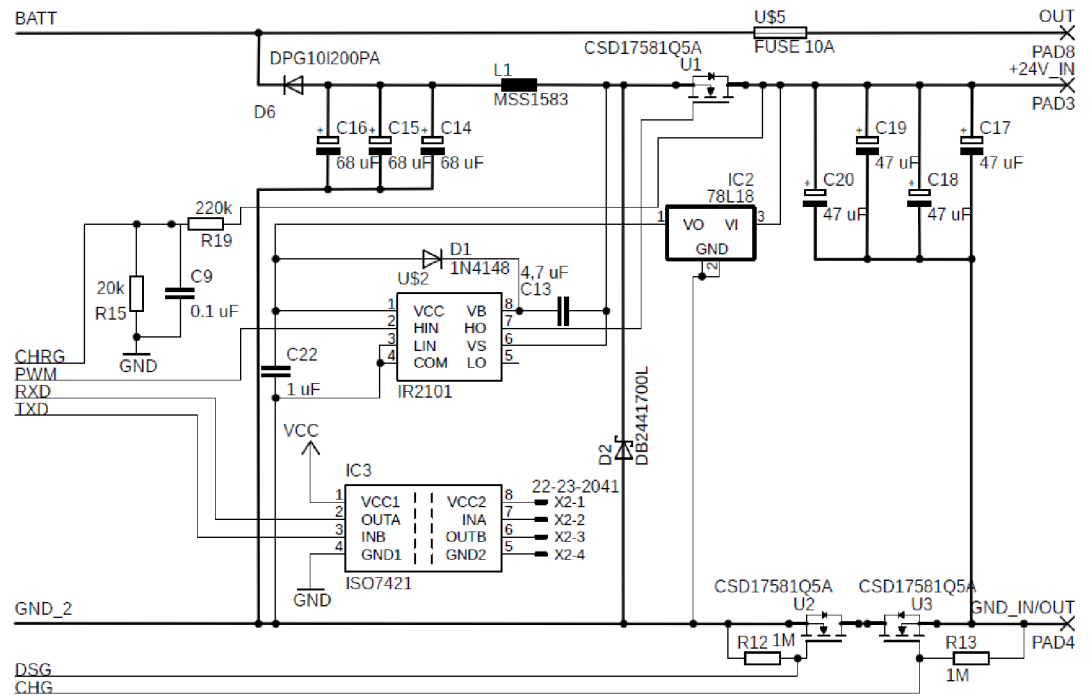
Obrázek 9.4 Schéma obvodu inteligentní baterie (část 2)
