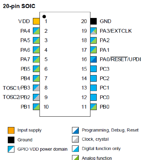
Obrázek 5.4 Rozložení pinů mikrokontroleru [14]
