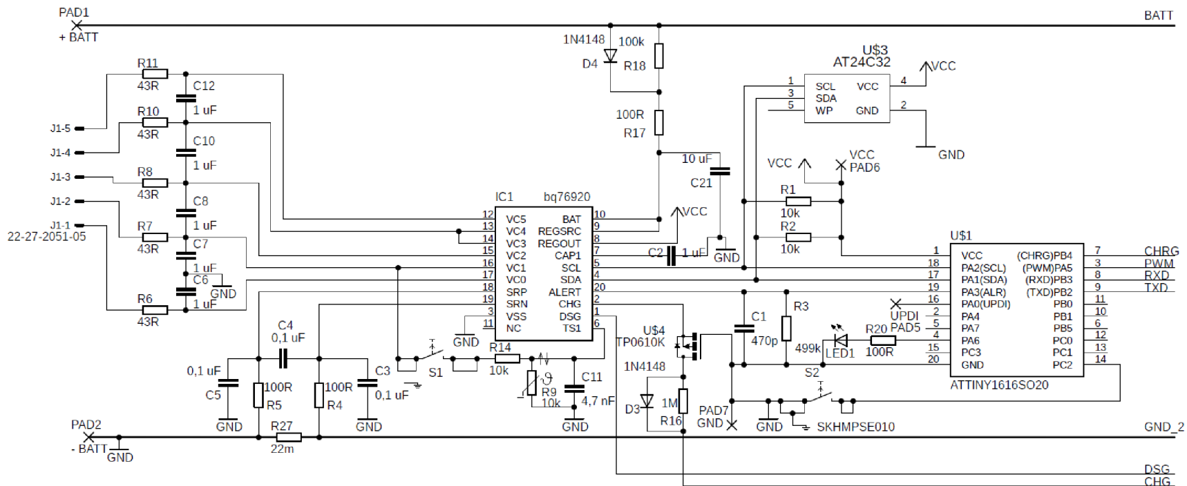
Obrázek 9.3 Schéma obvodu inteligentní baterie (část 1)
