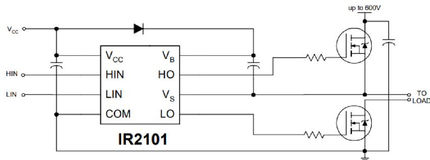
Obrázek 5.8 Zapojení high-side driveru [20]
