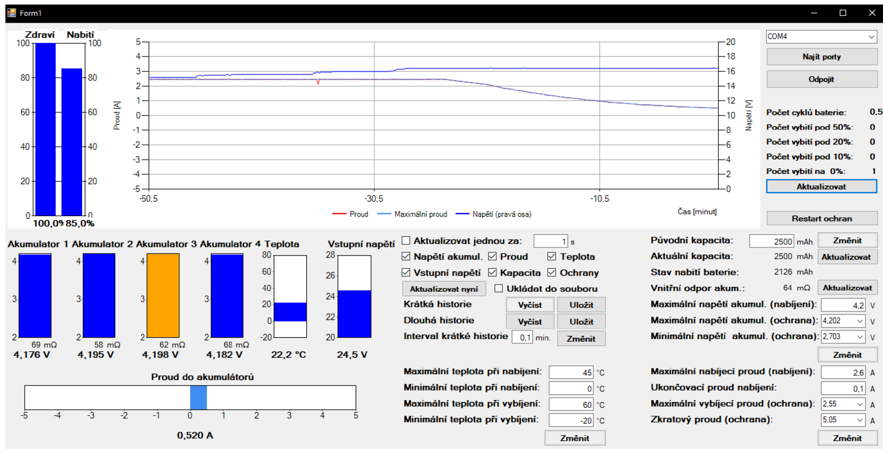
Obrázek 9.5 Počítačová aplikace
