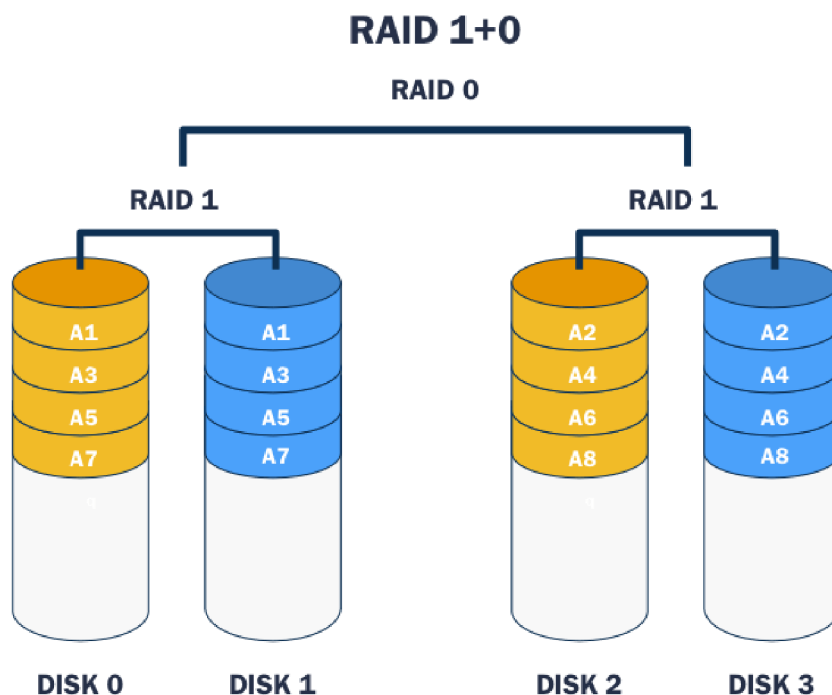
Obr. 13: Raid 10 (Zdroj: 9)
