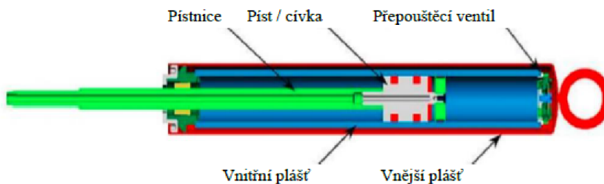
Obrázek 2.6: Dvouplášťový MR tlumič, převzato z [6]
