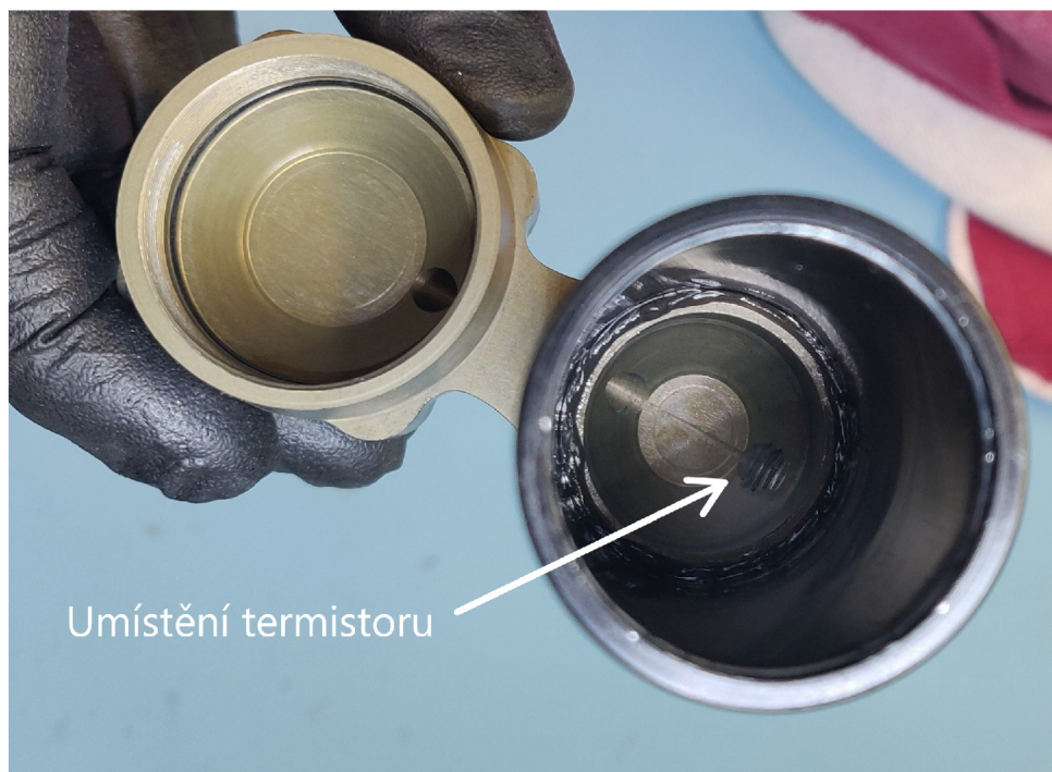
Obrázek 3.2: Umístění termistoru
