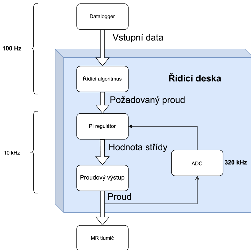
Obrázek 3.5: Vývojový diagram
