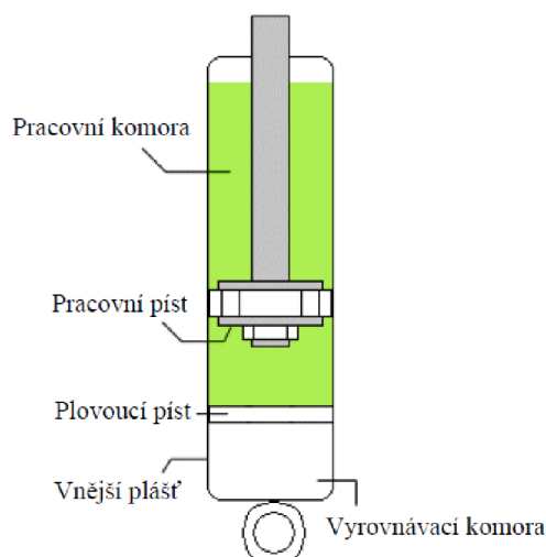
Obrázek 2.3: Řez jednoplášťovým teleskopickým tlumičem, převzato z [4]
