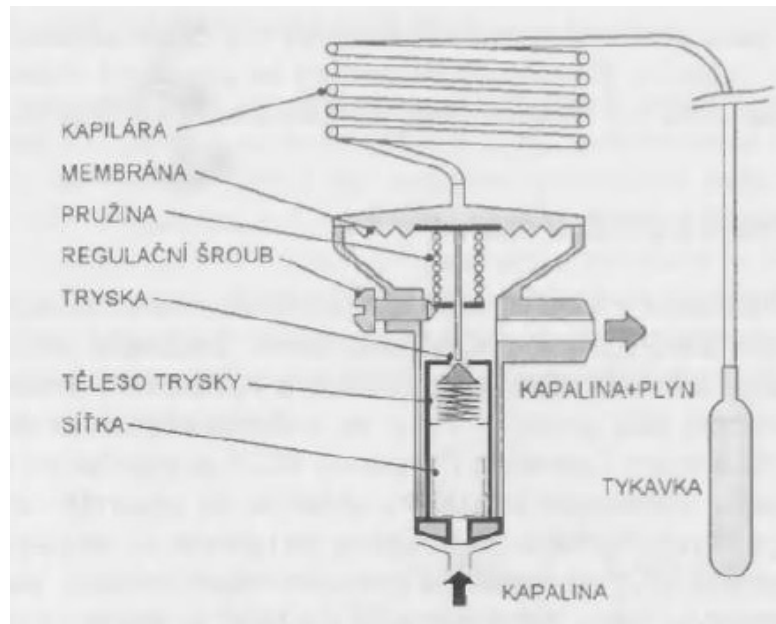
Obr. 9. Schéma TEV [11]
