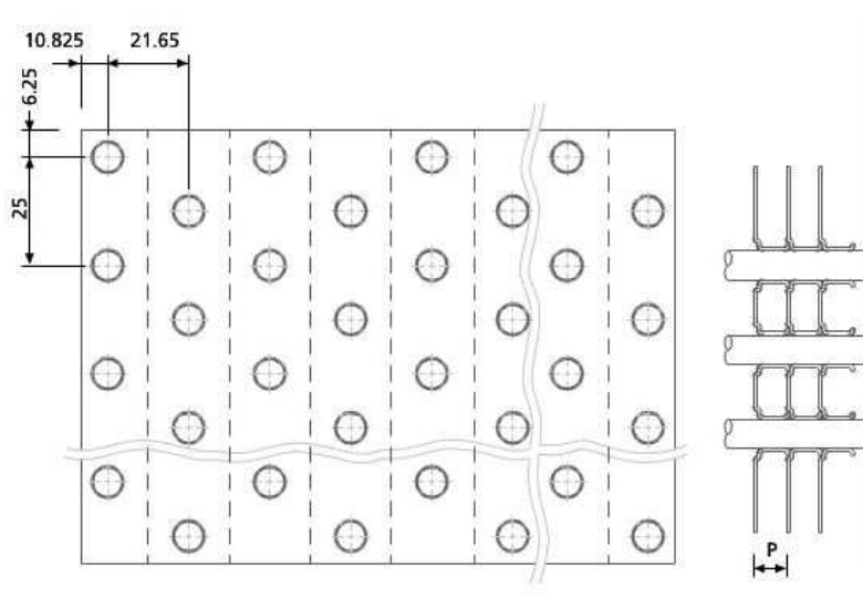
obr. 11.6. náčrt žebra výměníku
