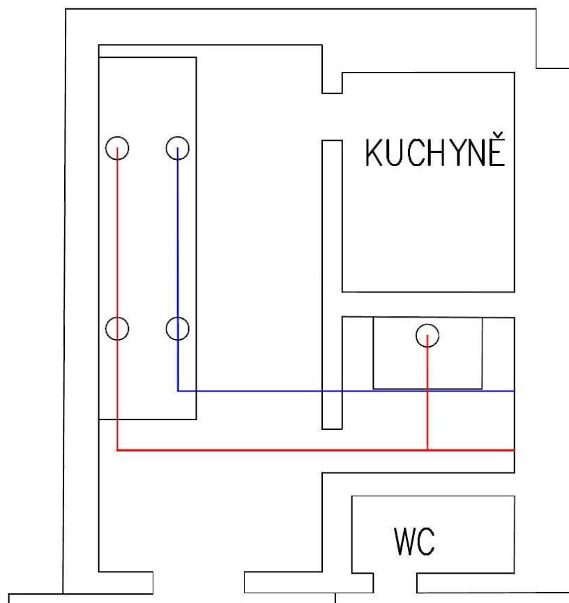
obr.11.3. prostorové uspořádání v kuchyni
