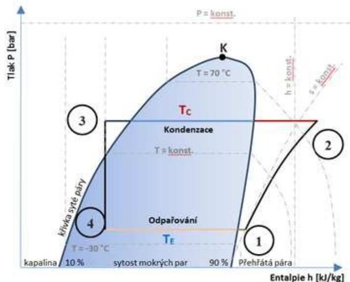
Obr. 1. Rankin - Clausiův cyklus TČ [15]
