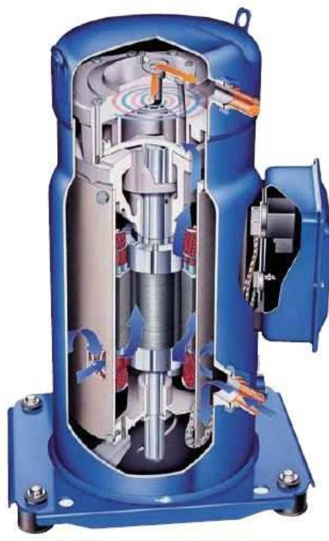
obr.13.1. řez kompresoru SZ
