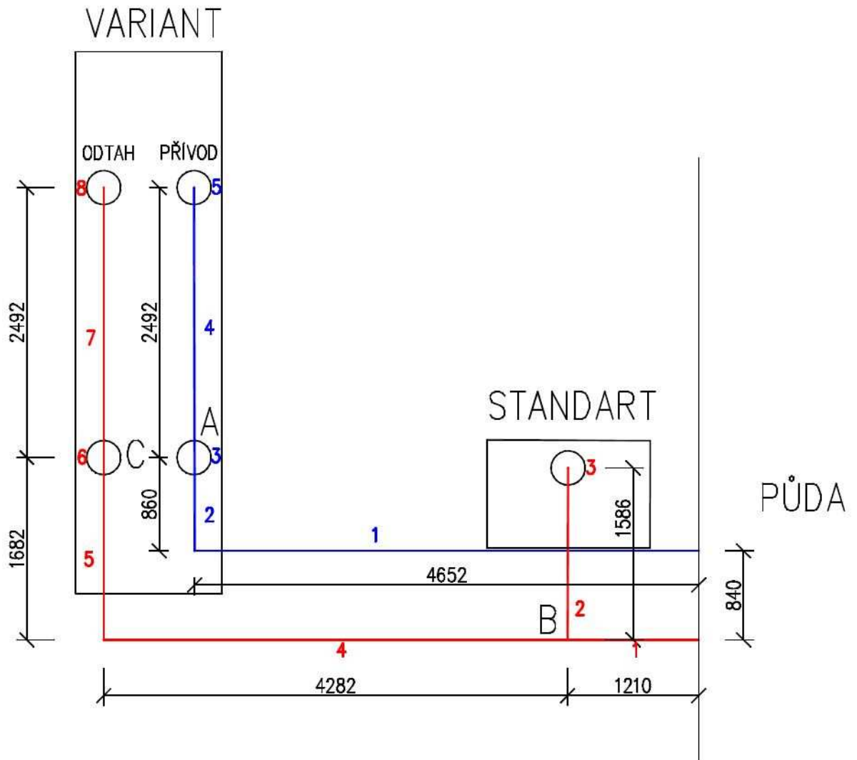
obr.11.4. zobrazení úseků a uzlů potrubí
