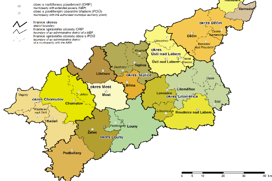
Obrázek 1 Okresy Ústeckého kraje
