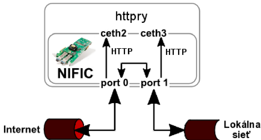
Obrázok 4.6: Schéma zapojenia manažéra prístupu na webové stránky
