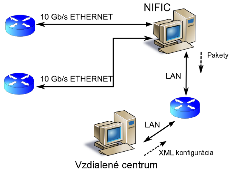
Obrázok 3.3: NIFIC ako vzdialene konfigurovaný filter
