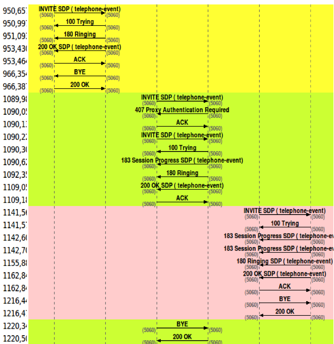
Obrázok 5.2: Ukážka grafu zachytených VoIP hovorov
