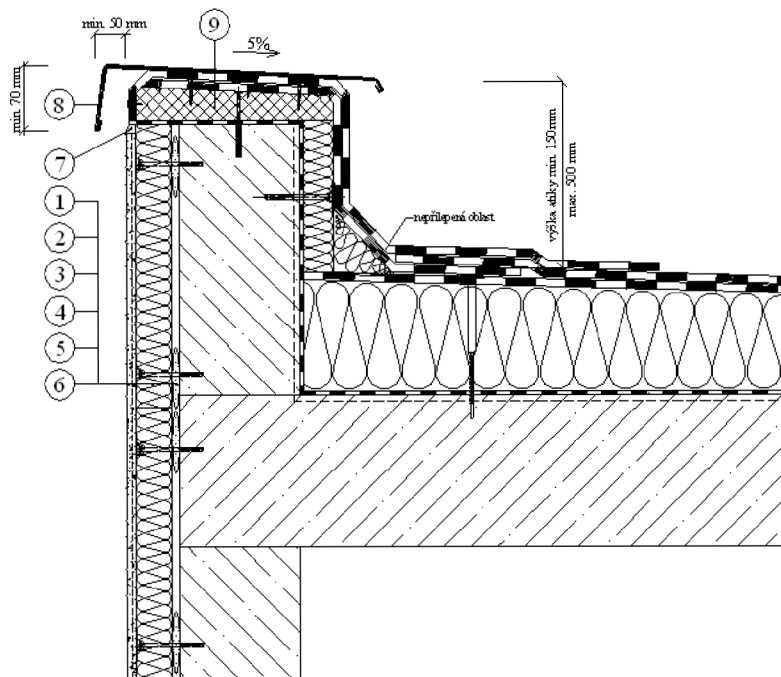
Obr.11 – Detail zateplení u atiky
