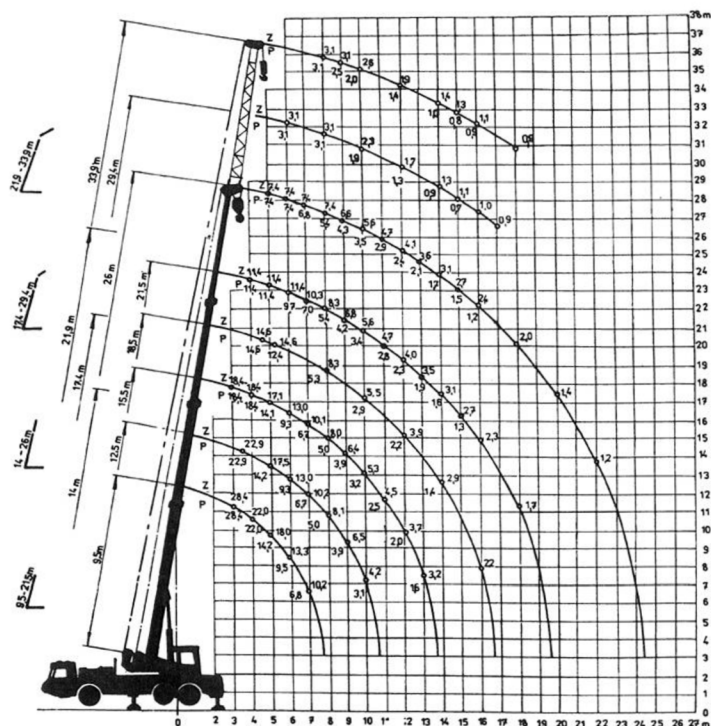
Obr.31 Graf nosnosti a výložení autojeřábu Tatra AD28
