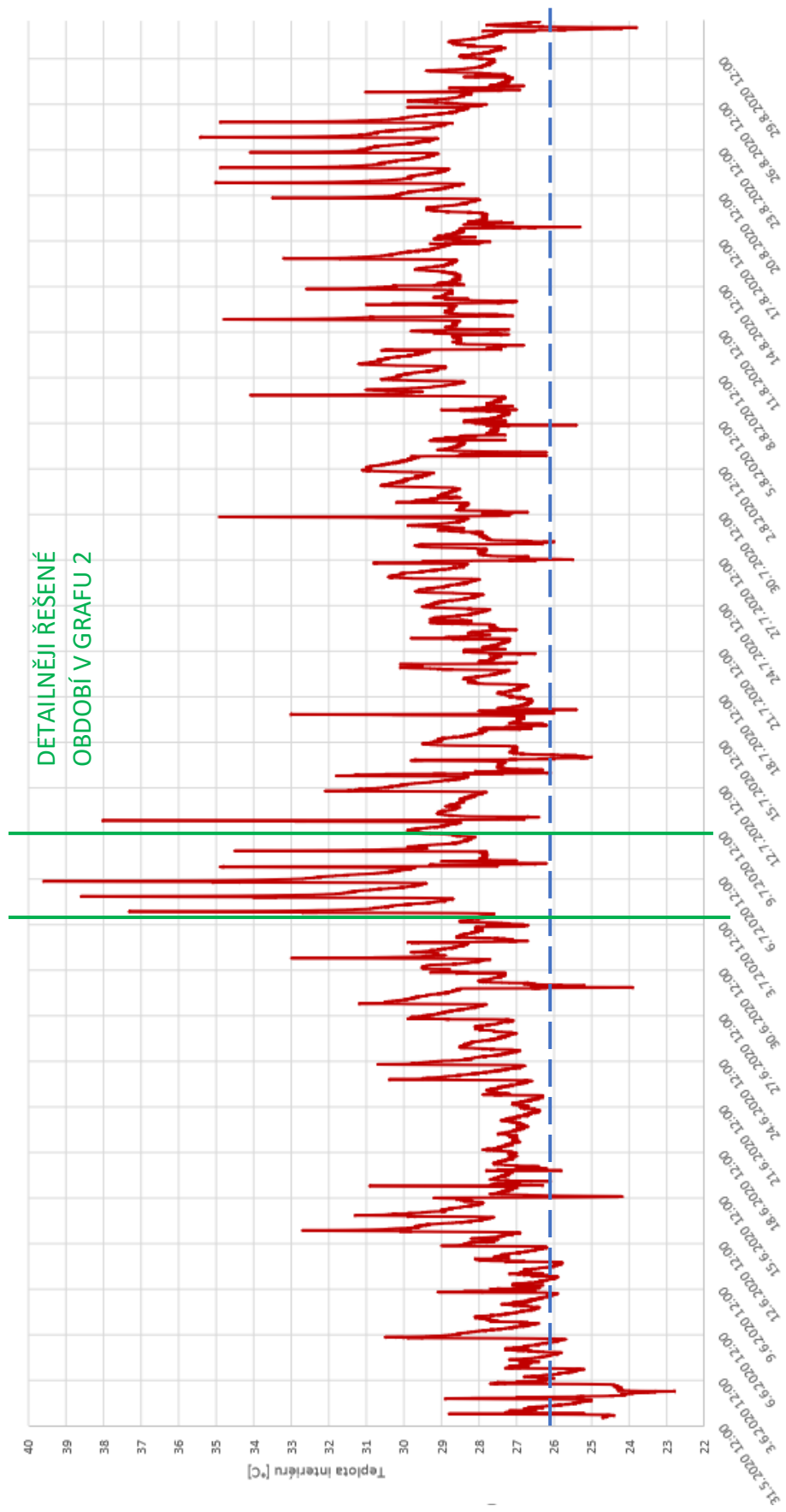
Graf 1 - průběh teplot vnitřního vzduchu v místnosti 3.07 v období od 1.6. do 31.8.2020
