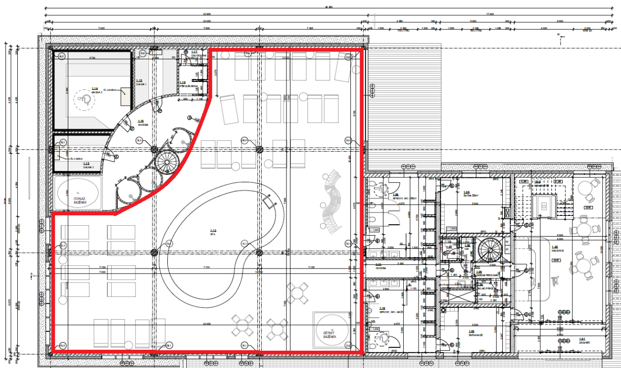
Obr. 1 Půdorys prvního podlaží Wellness Čeladná s označením řešené oblasti
