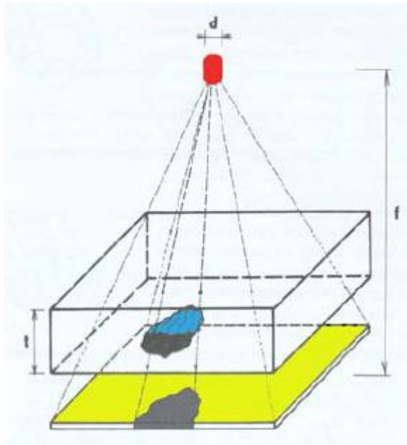
Obrázek 2 : Centrální projekce
