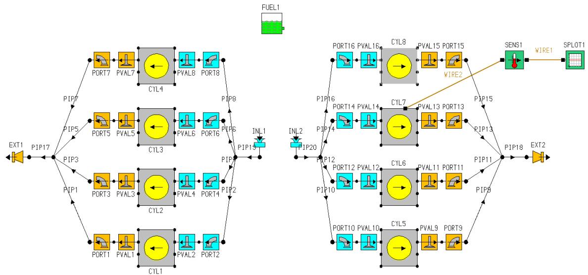
Obr. 62 Termodynamický model motoru
