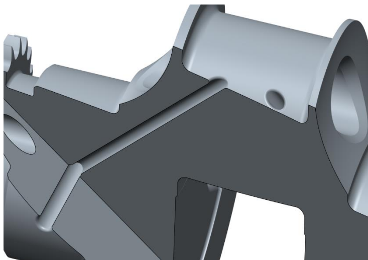
Obr. 23 Mazání ojnicího čepu
