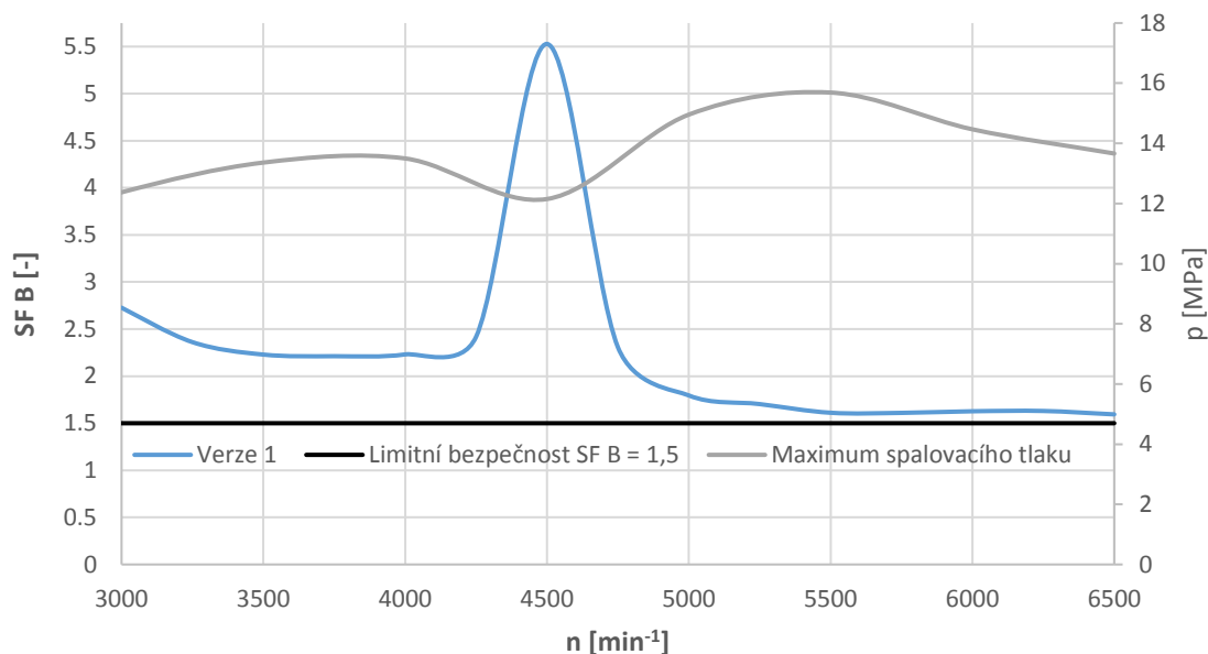
Obr. 58 Koeficient bezpečnosti vůči mezi trvalé pevnosti varianty 1
