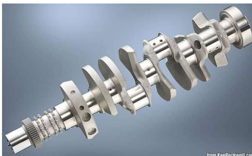
Obr. 3 Klikový hřídel motoru S65B40 [3]
