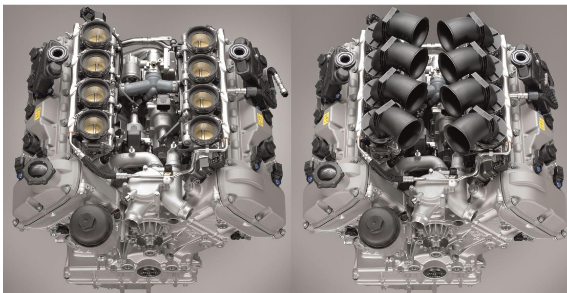
Obr. 7 Škrticí klapky a svody sání motoru S65B40 [2]
