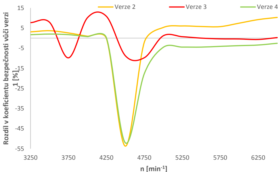
Obr. 60 Poměrný rozdíl v bezpečnosti vůči sériovému pořadí zážehů
