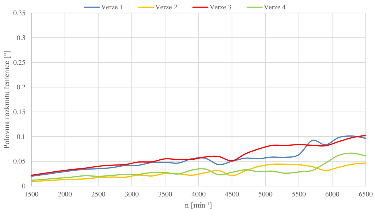
Obr. 106 3,5. řád harmonické složky kmitání řemenice
