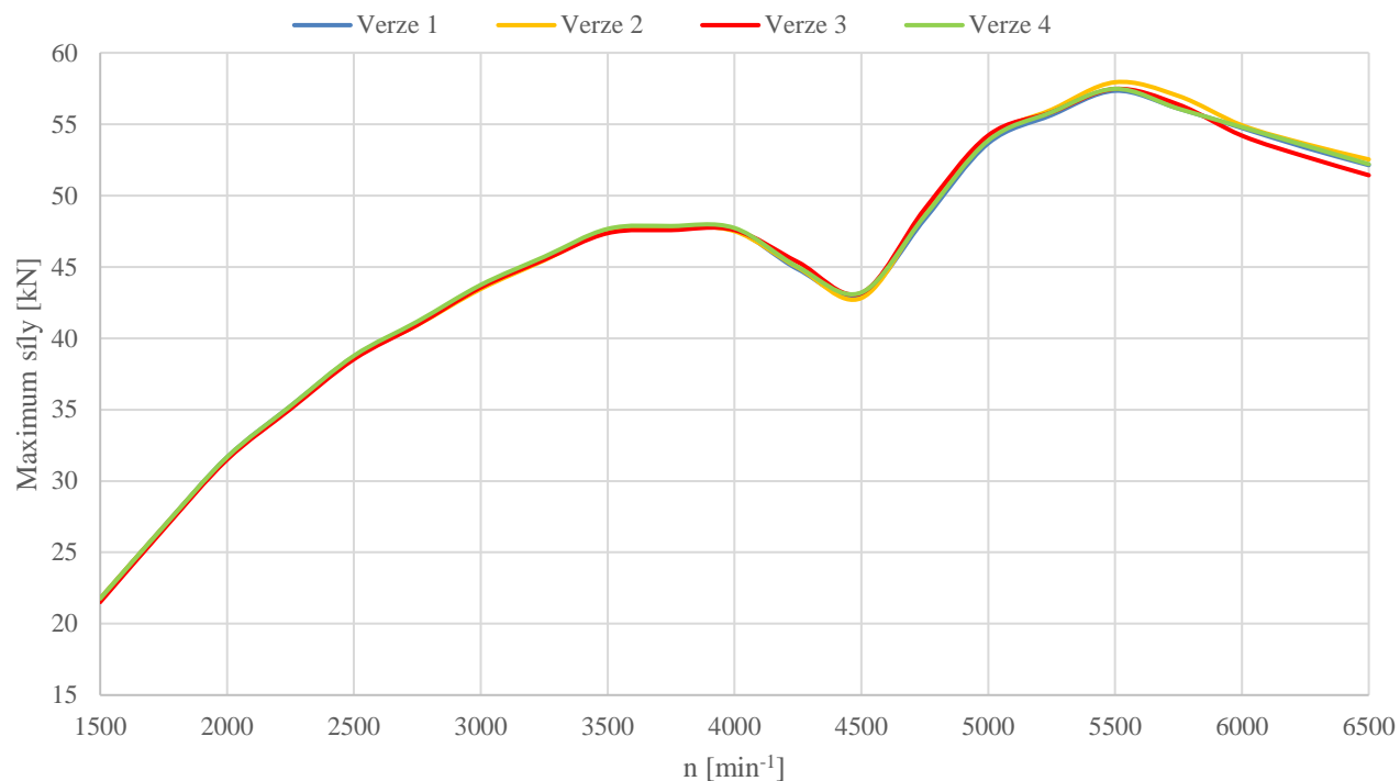
Obr. 92 Zatížení pátého hlavního ložiska
