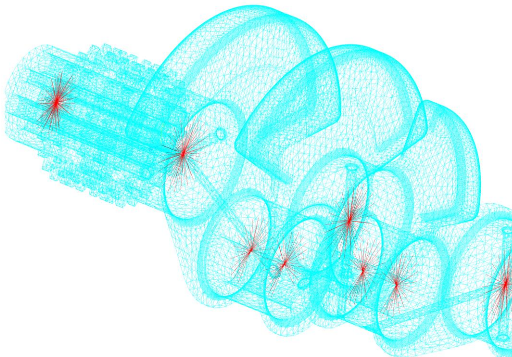
Obr. 37 Prutové výztuhy ve struktuře klikového hřídele
