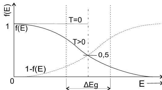
Obr. 2.4: Funkce pravděpodobnosti f(E) a 1 - f(E) [1]
