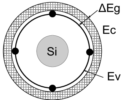
Obr. 2.1: Atom křemíku se znázorněnými energetickými hladinami
