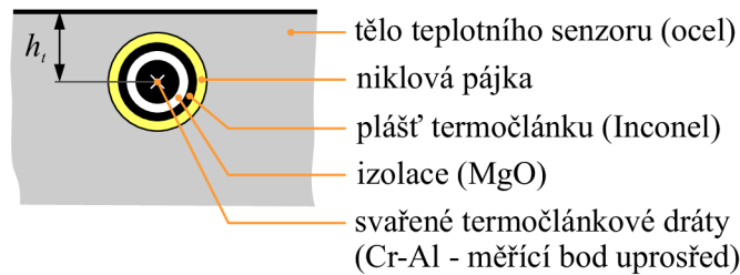
Obrázek 3.19: DROT - schématické znázornění modelu vrtaného teplotního senzoru se zapájeným termočláčkem pro inverzní úlohu vedení tepla
