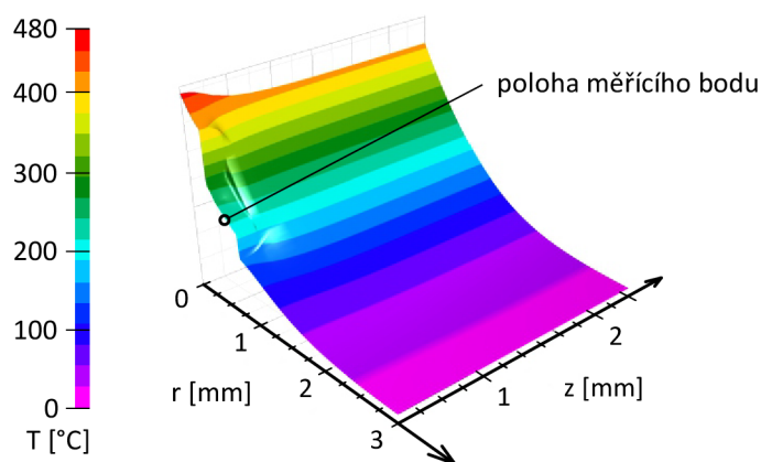
Obrázek 3.20: Ovlivnění teplotního pole ve válci přítomností termočláčku modelu DRILL. Hloubka termočláčku h_t = 0,5\text{mm}
