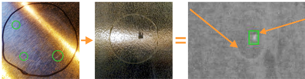
Obrázek 4.14: Povrch senzoru po přebroušení (vlevo), po vyválcování 15 svítků (uprostřed), obraz jeho otisku ve válcovaném materiálu v detekčním systému (vpravo)
