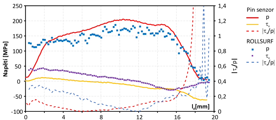
Obrázek 4.19: H2 - kontaktní napětí ve válcovací mezeře, poměr |\tau_x/p| , porovnání senzoru ROLLSURF a pin senzoru
