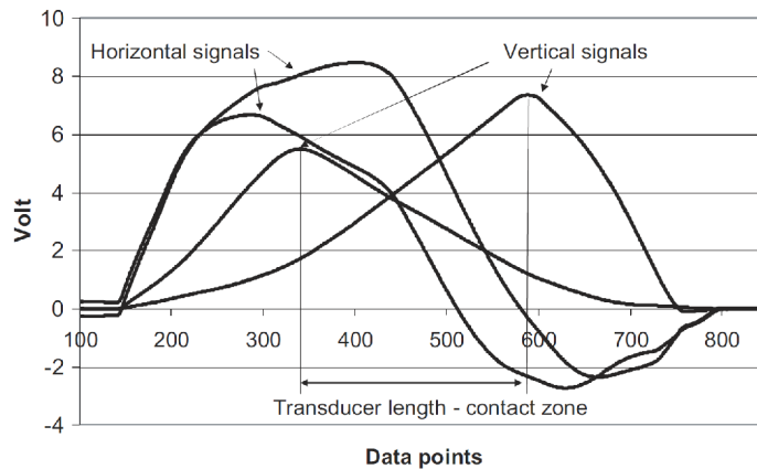
Obrázek 2.10: Výstupní signál z tenzometrů během průchodu snímače válcovací mezerou [48]
