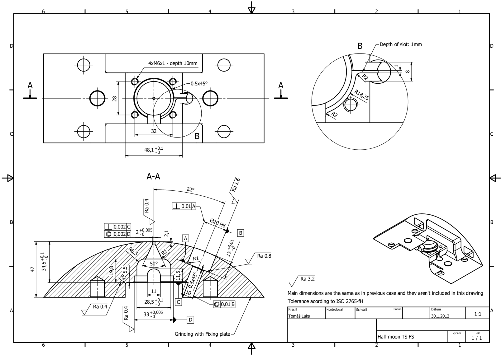
Obrázek A.13: Dutina ve válci pro pin senzor
