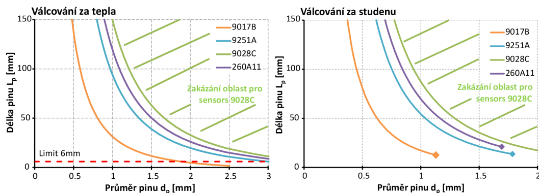
Obrázek 3.36: Limitace velikosti pinu senzoru na základě mechanických limitů snímačů pro extrémní případy válcování
