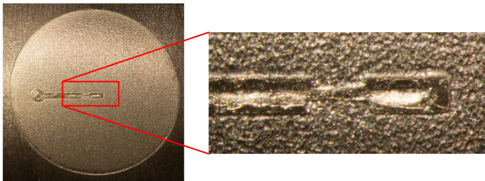
Obrázek 4.26: Propad pájky nad termočlánkem
