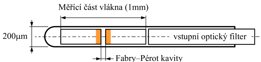
Obrázek 2.12: Schématická ukázka měřící části optického vlákna
