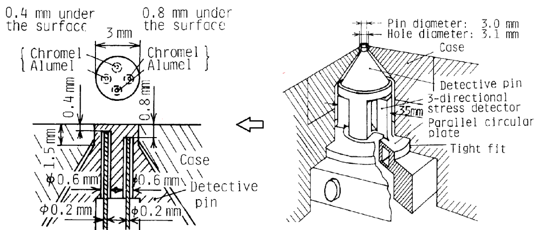
Obrázek 2.14: Termočlánek instalovaný v pin senzoru [36]
