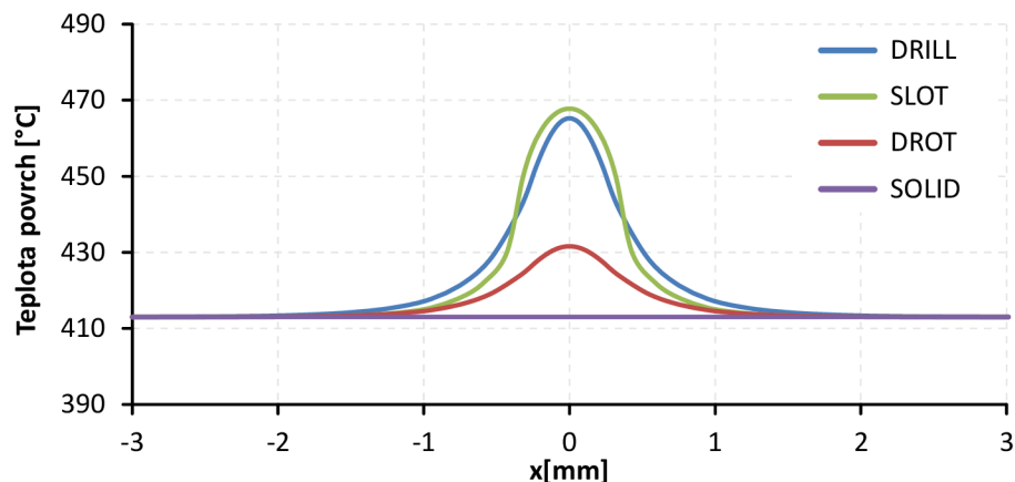
Obrázek 3.21: Teplota povrchu nad termočláčkem pro různé typy senzorů. Hloubka termočláčku h_t = 0,5\text{mm}
