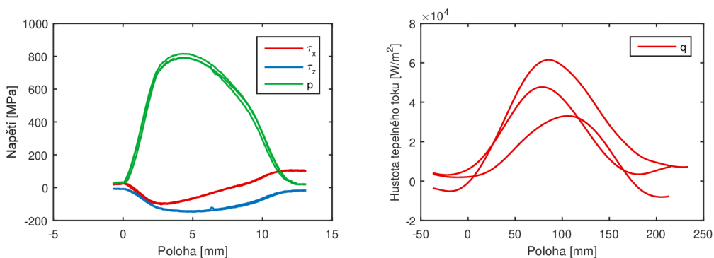
Obrázek C.1: C1: napětí v kontaktu a hustota tepelného toku ve válč. mezeře
