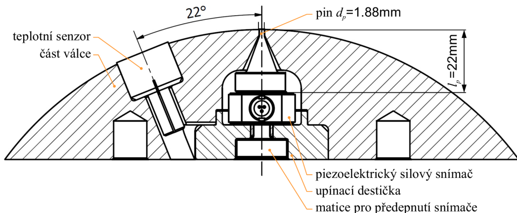
Obrázek 3.34: Teplotní senzor a pin senzor ve válci zobrazený v řezu
