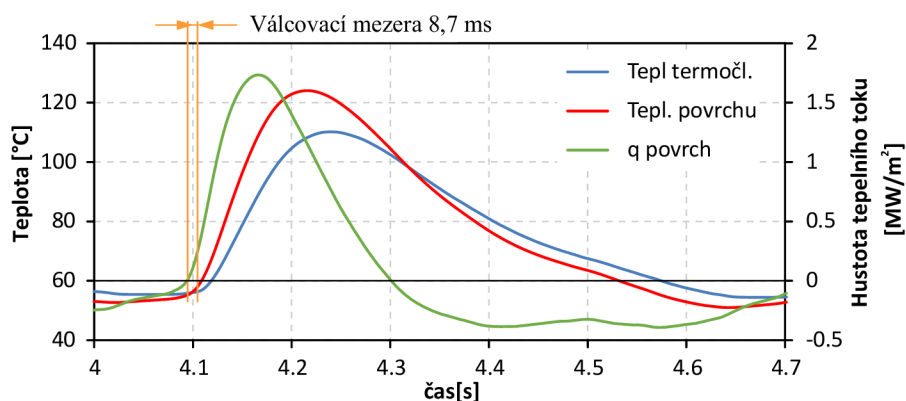
Obrázek 4.11: Svitek č.1, senzor S4, srovnání teplot a hustoty tepelného toku s velikostí válcovací mezeře
