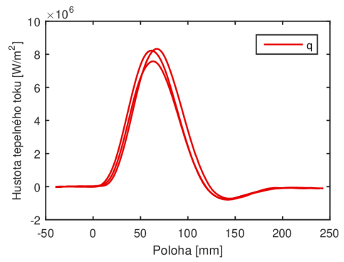
Obrázek C.16: H7: napětí v kontaktu a hustota tepelného toku ve válč. mezeře
