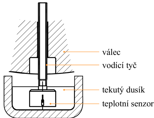
Obrázek 3.5: Etapa II - Instalace pomocí tekutého dusíku
