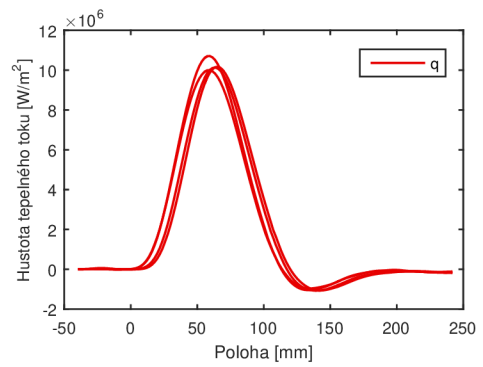
Obrázek C.17: H8: napětí v kontaktu a hustota tepelného toku ve válč. mezeře
