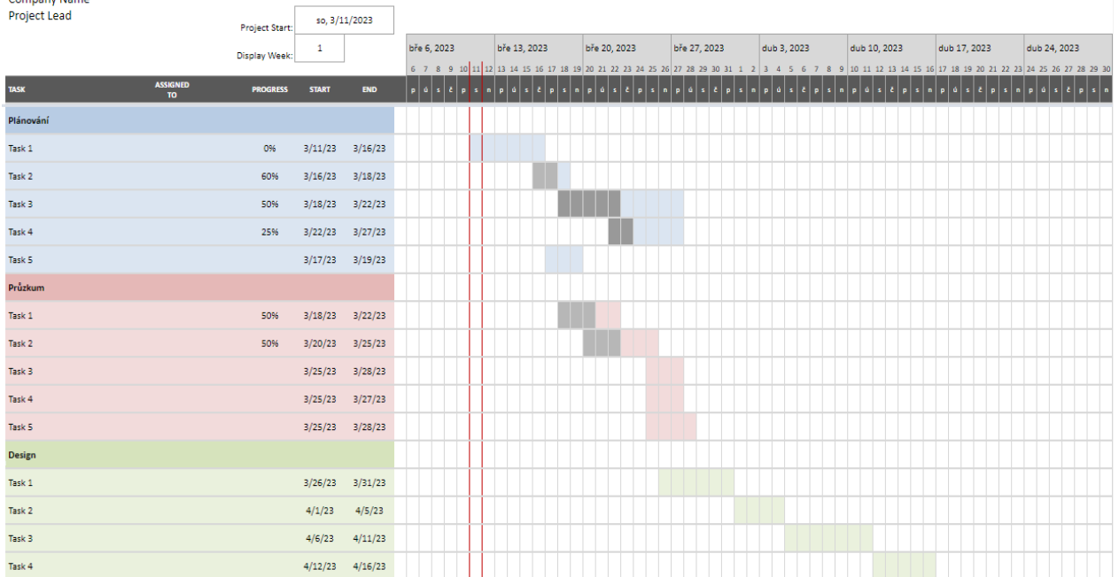
Obrázek 5: Ganttův diagram
