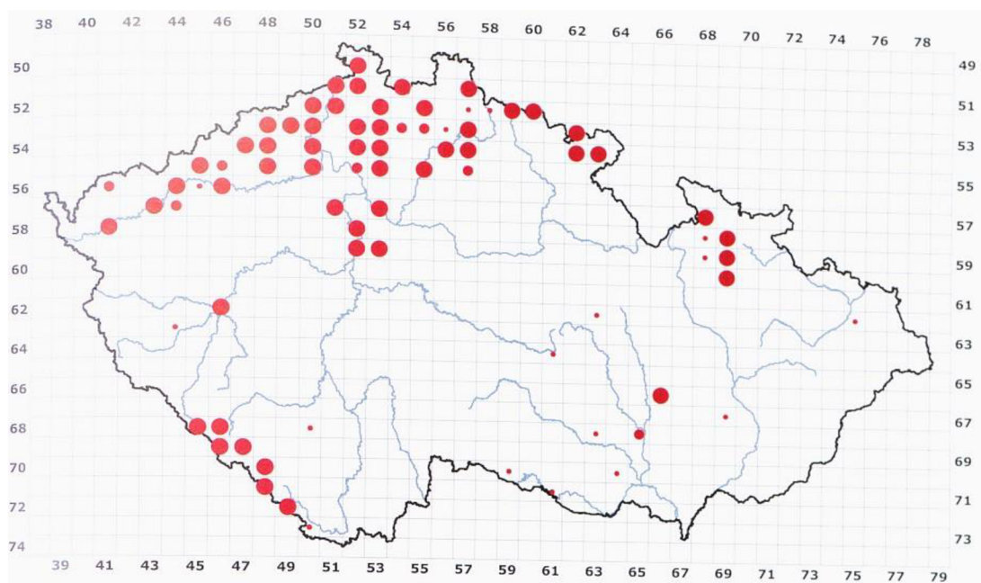
Obrázek 4: Hnízdni rozšíření sokola stěhovavého v kvadrátové síti 12 x 11,1 km v letech 2014–2017 převzato z Šťastného et al. (2021)
