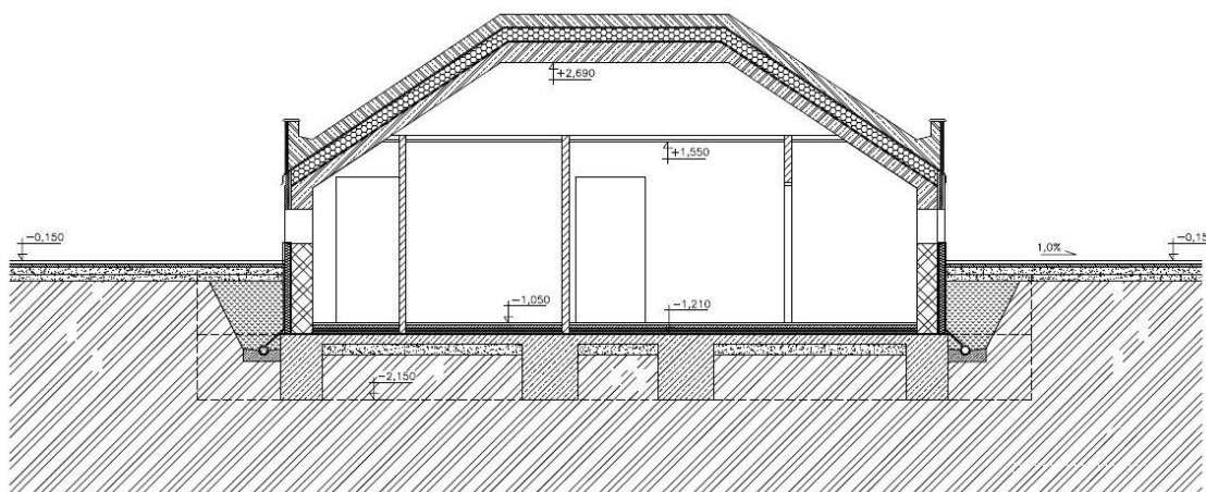
SCHEMA - HRUBÁ VRCHNÍ STAVBA ŘEZ B-B'
