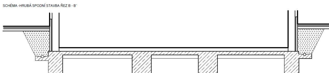
Obr. 7 Základy [7]
