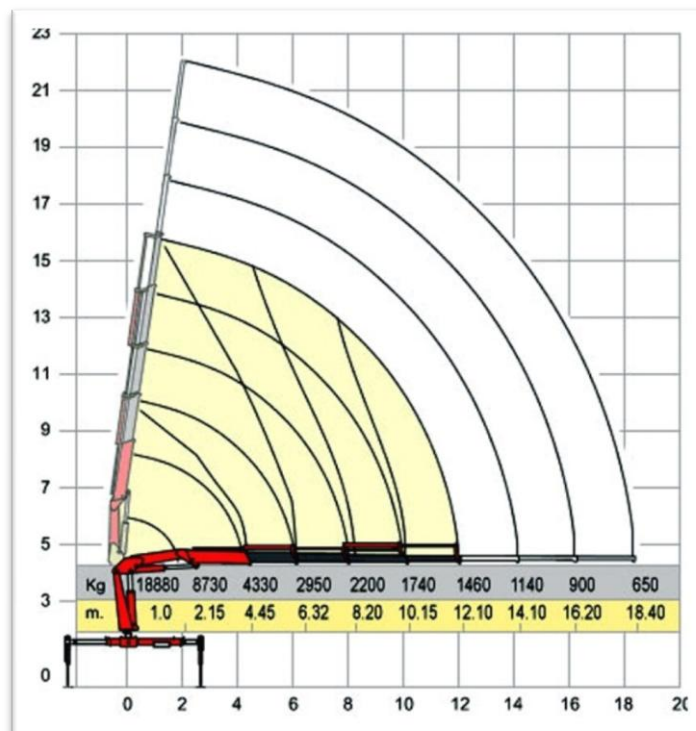
Obr. 21 Hydraulická ruka Amco Verba [21]
