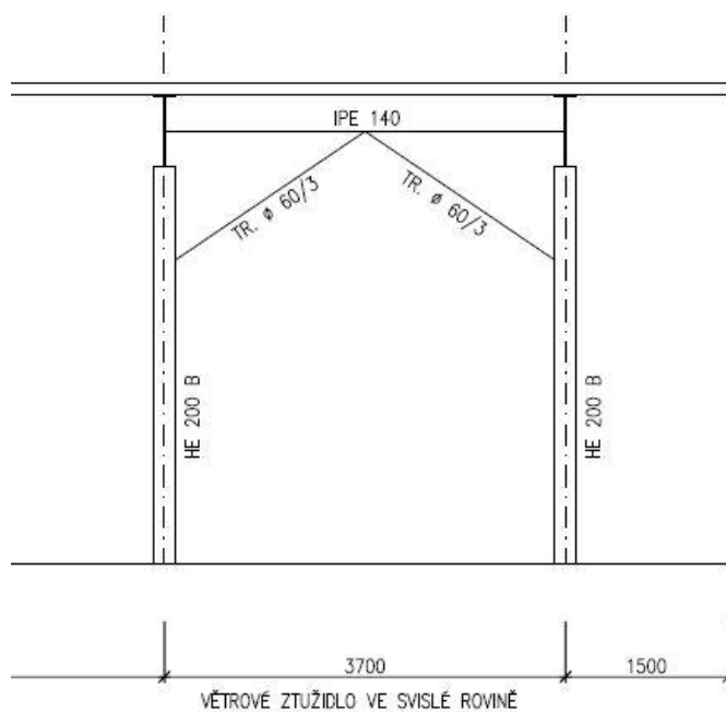
Obr. 42 Pohled na větrové ztužidlo ve svislé rovině [42]
