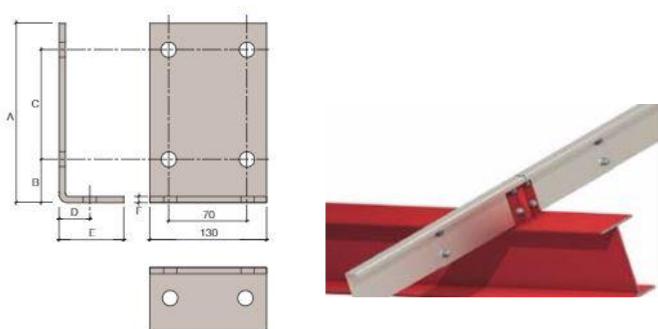
Obr. 101: profily 142 - 262 šroubované kotevní botky
