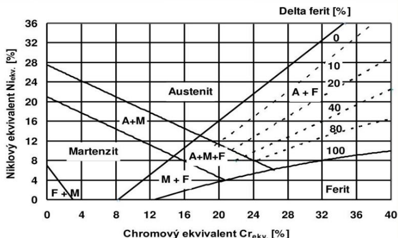
Obr. 5 Schaefflerův diagram [3].
