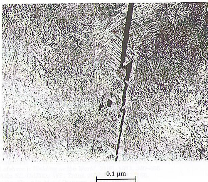
Obr. 15 Vodíková trhлина [8].
