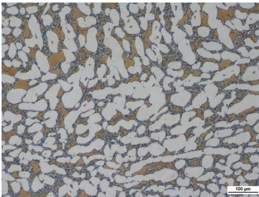
Obr. 4 Duplexní ocel po kování - 100 x zvětšeno (hnědá fáze - ferit, bílá fáze - austenit, drobné částice - sigma fáze) [12].
