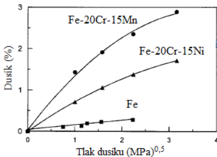
Obr. 7 Rozpustnost dusíku ve slitinách Fe při 1600 °C v závislosti na tlaku N 2 nad taveninou [11].
