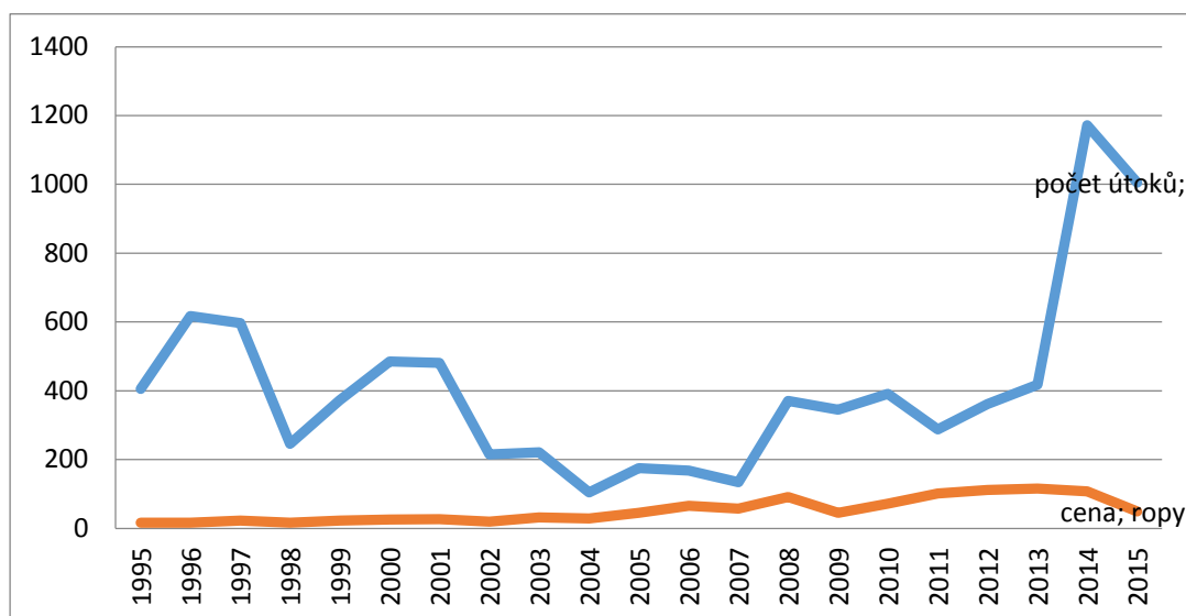
Obrázek 4 Grafické znázornění sbíraných dat
