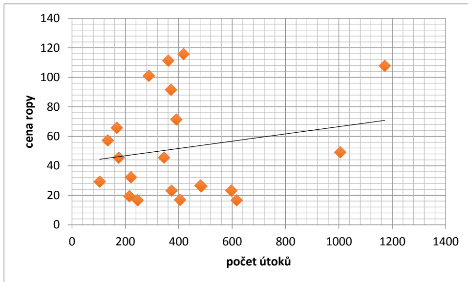
Obrázek 5 Grafické vyjádření korelačního koeficientu
