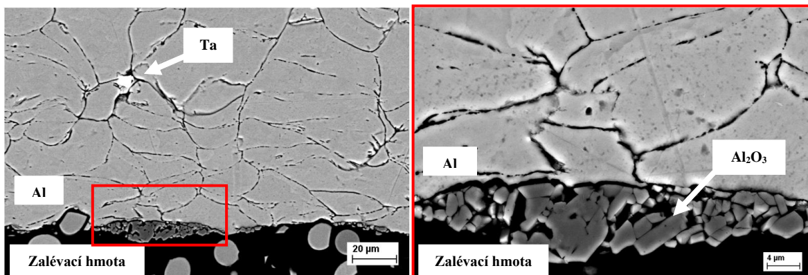
Obrázek 32 - Elektronová mikroskopie rozhraní BSE mod- vlevo zvětšeno 500x, vpravo zvětšeno 2300x
