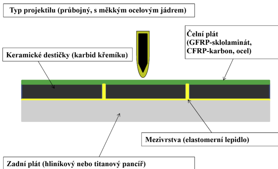
Obrázek 1 - Schéma keramického vícevrstvého systému balistické ochrany
