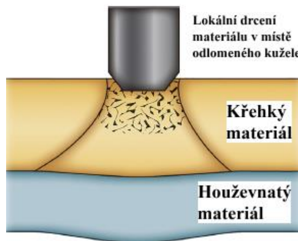
Obrázek 22 - Drcení materiálu
