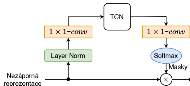
Obrázek 4.3: Schéma separačního modulu, jehož vstupem je nezáporná reprezentace směsi mluvcích.
