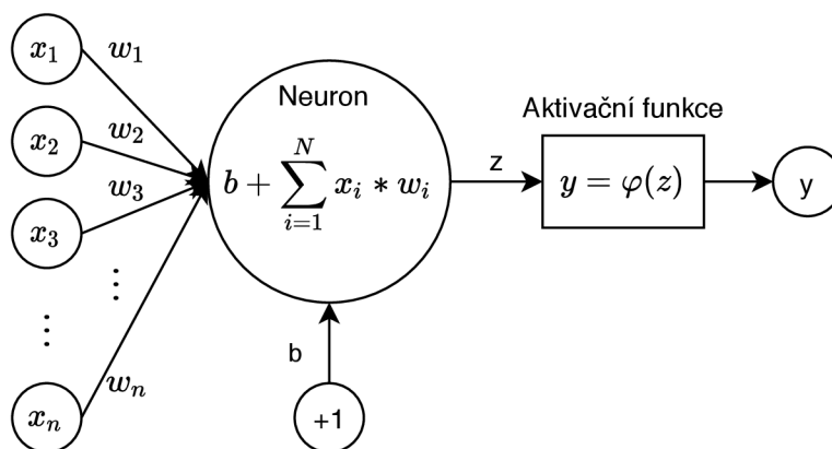
Obrázek 3.3: Schéma umělého neuronu.
