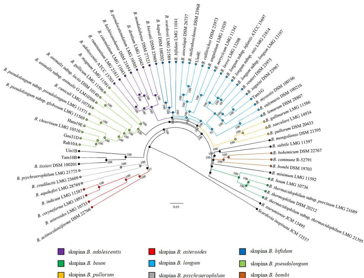
Obrázek 3: Fylogenetický strom rodu Bifidobacterium zobrazující devět fylogenetických skupin, založený na konkatenci odvozených aminokyselinových sekvencí 232 základních genů Goo31D, Ham19E, Rab10A, Tam1G, Uis4E a Uis1B bootstrap (Lugli et al. 2018)
