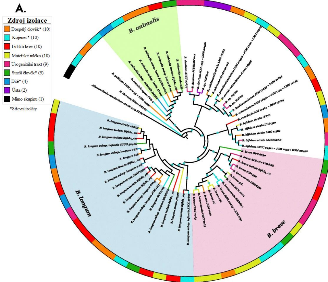
Obrázek 4: Fylogenetický vztah kmenů Bifidobacterium odvozených od člověka na základě 107 markerových genů. Významné druhy jako B.longum, B. breve a B. animalis jsou vystínovány různými barvami. Vnější kroužek představuje různé zdroje izolace bifidobakterií (Rodriguez & Martiny, 2020)
