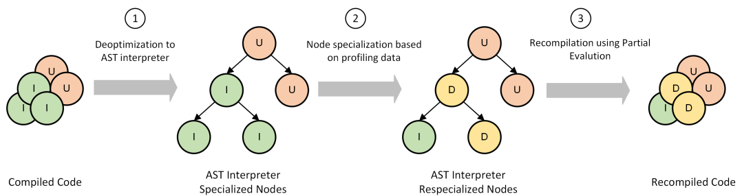
Obrázek 16: Jestliže spekulace stability stromu je porušena, dochází k deoptimizaci, strojový kód je zahozen a AST strom se interpretuje (1). Uzly se opět specializují na základě profilujících dat (2), a jakmile jsou podmínky pro JIT kompilaci znovu splněny, dochází k další kompilaci do strojového kódu (3) [25]
