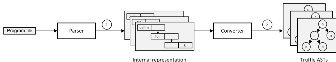
Obrázek 17: Architektura interpretu
