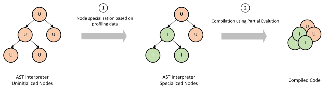
Obrázek 15: Na základě profilujících dat se uzly specializují (1). Jakmile je strom stabilní a počet volání metody překročí hranici pro JIT kompilaci, je na specializovaný strom nejprve aplikována PE a poté je přeložen do strojového kódu (2) [25]
