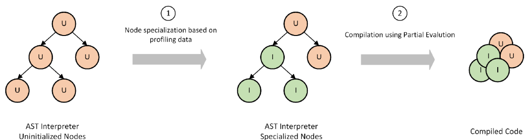
Obrázek 15: Na základě profilujících dat se uzly specializují ①. Jakmile je strom stabilní a počet volání metody překročí hranici pro JIT kompilaci, je na specializovaný strom nejprve aplikována PE a poté je přeložen do strojového kódu ② [25]
