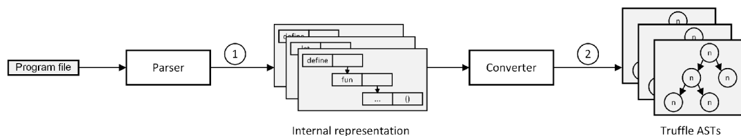
Obrázek 17: Architektura interpretu
