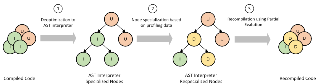
Obrázek 16: Jestliže spekulace stability stromu je porušena, dochází k deoptimizaci, strojový kód je zahozen a AST strom se interpretuje ①. Uzly se opět specializují na základě profilujících dat ②, a jakmile jsou podmínky pro JIT kompilaci znovu splněny, dochází k další kompilaci do strojového kódu ③ [25]
