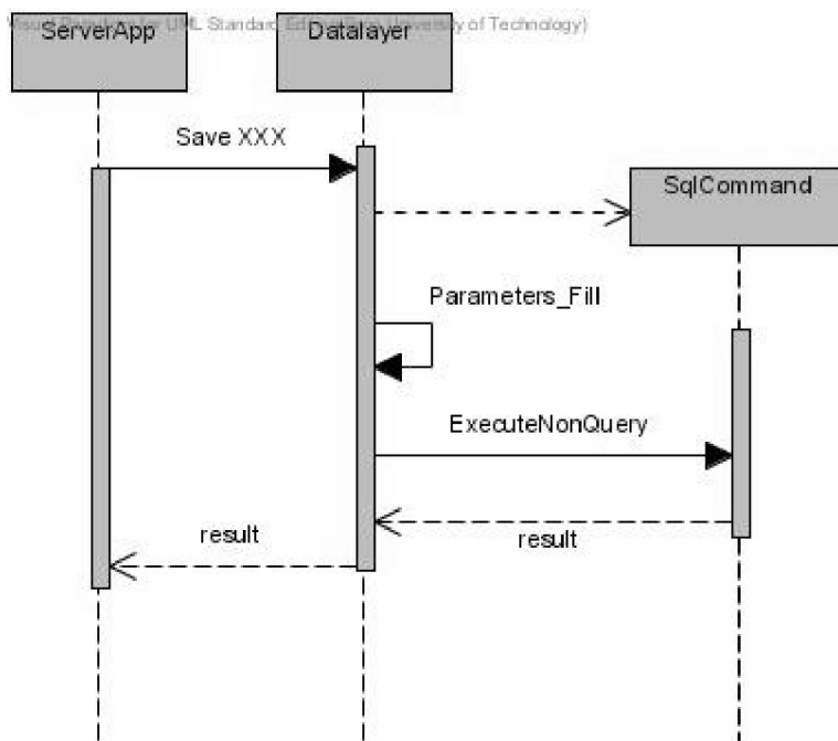
Obrázek 5.3 – Diagram sekvence operace Save XXX nad jediným záznamem
