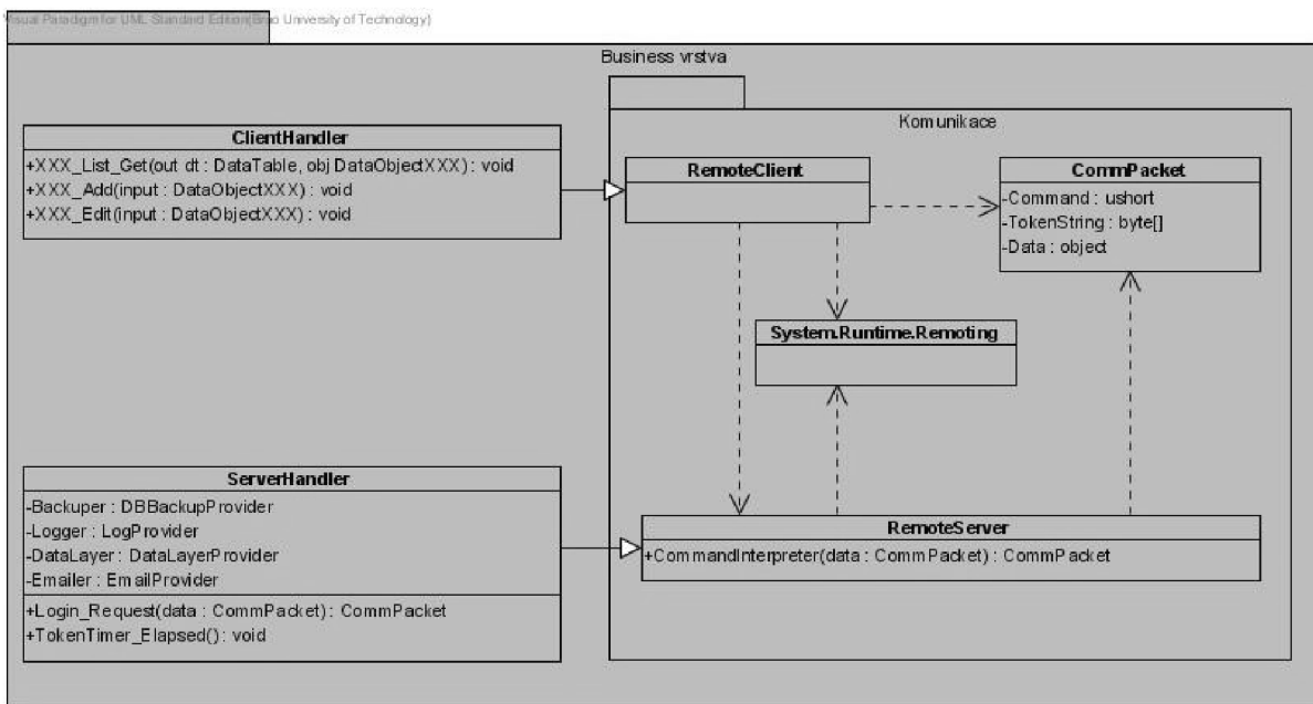
Obrázek 5.5 – Zjednodušený diagram návrhových tříd business vrstvy
