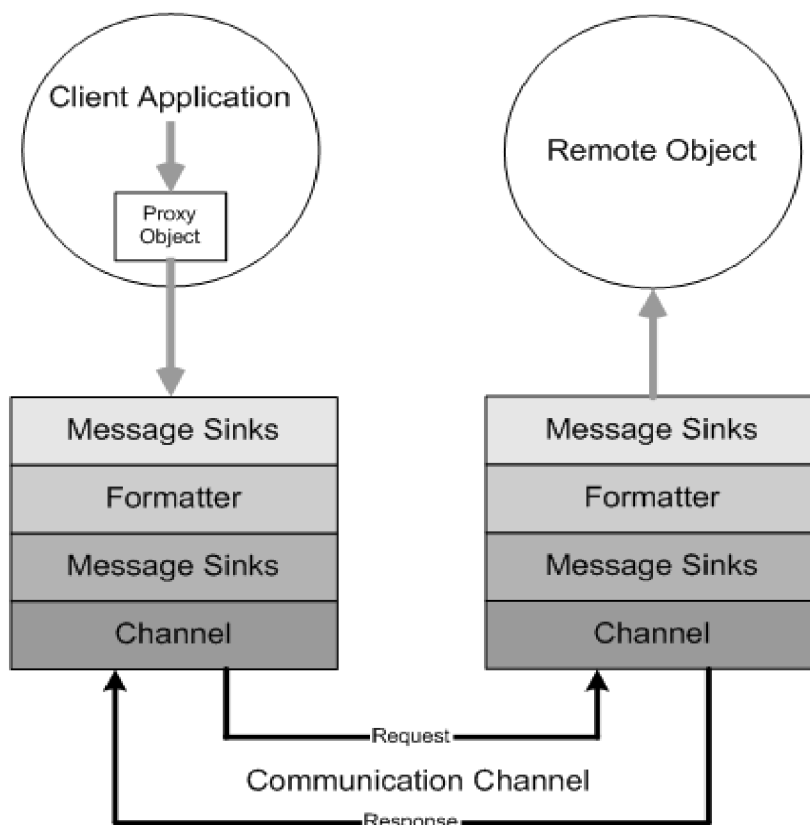
Obrázek 3.2 – Komunikace v .NET Remoting
