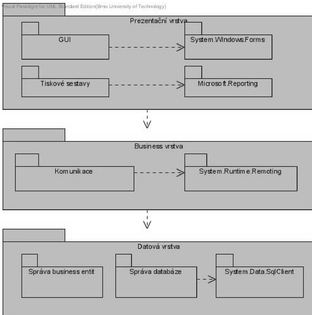
Obrázek 4.3 – Návrh architektury
