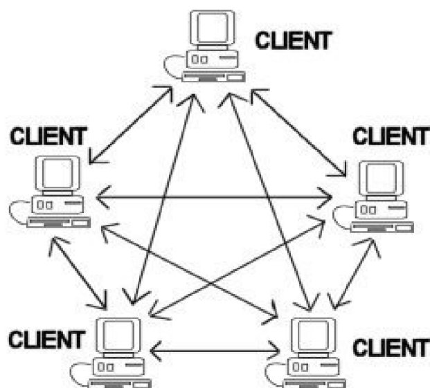
Obrázek 2.3 – Peer-to-Peer síť
