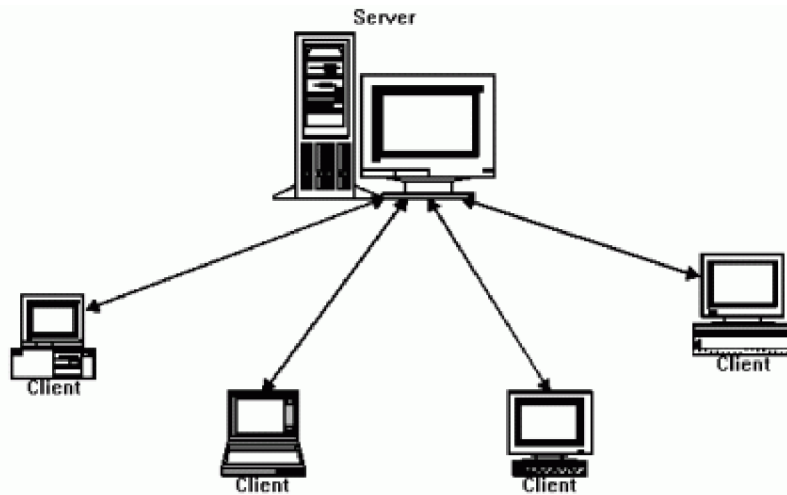
Obrázek 2.2 – Klient-Server
