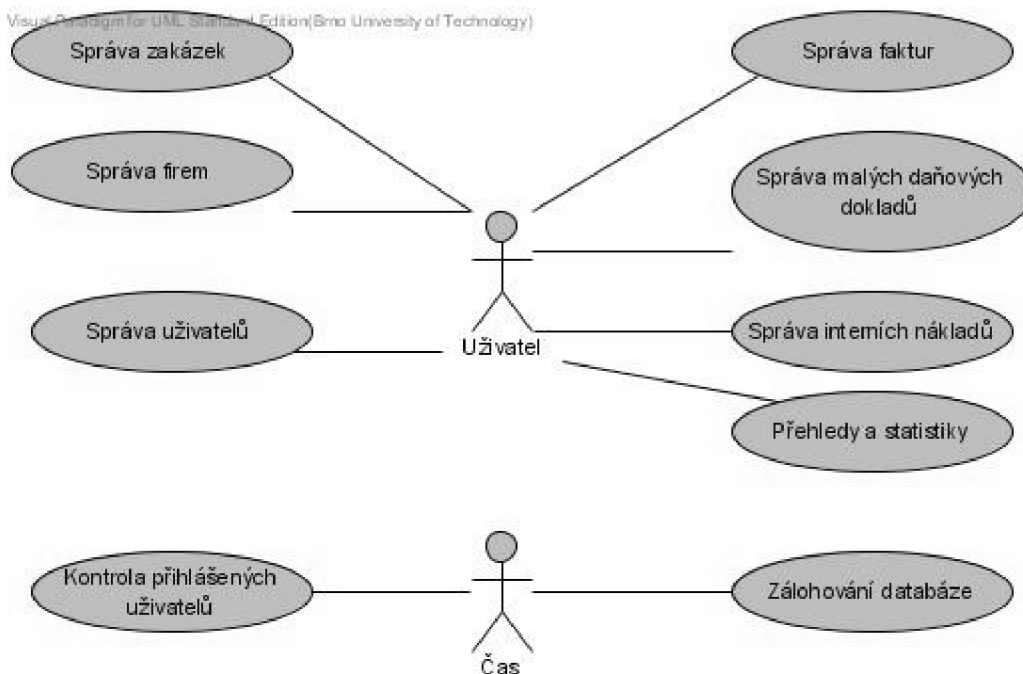
Obrázek 4.1 – Zjednodušený diagram případu užití systému
