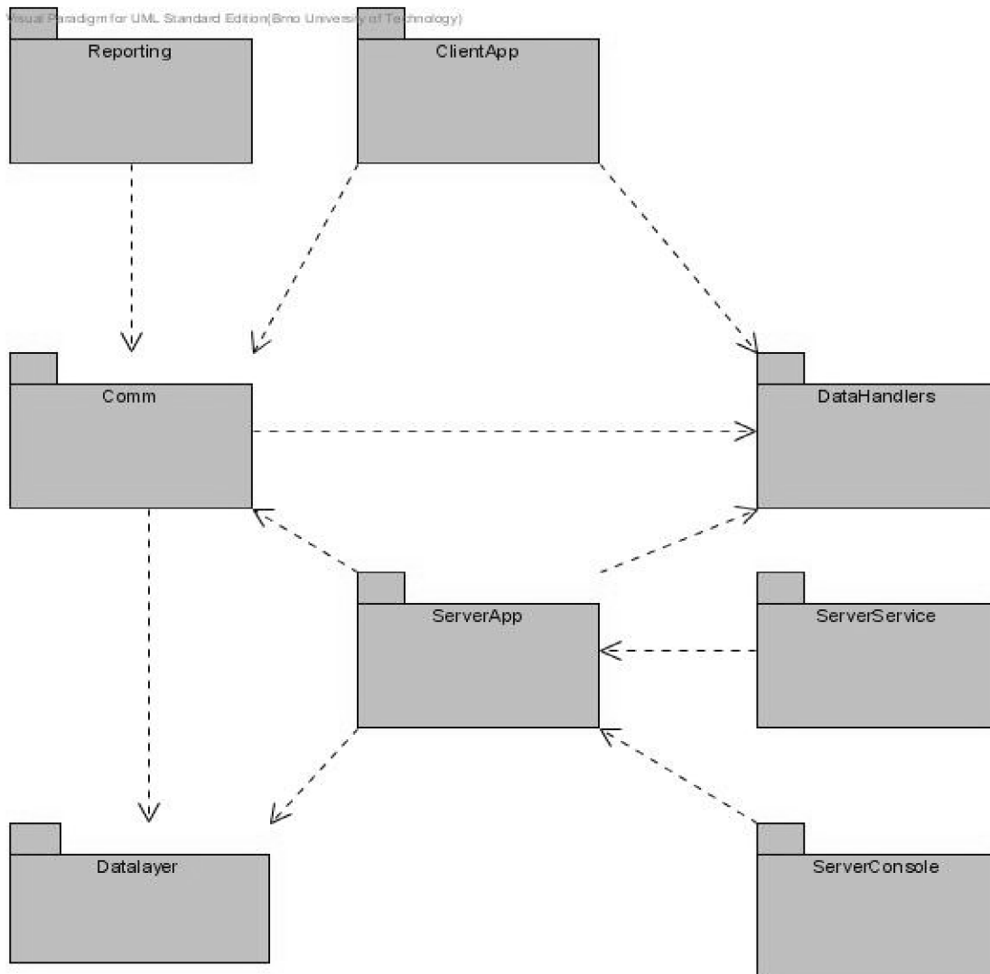
Obrázek 5.1 – Schéma logické závislosti aplikačních modulů
