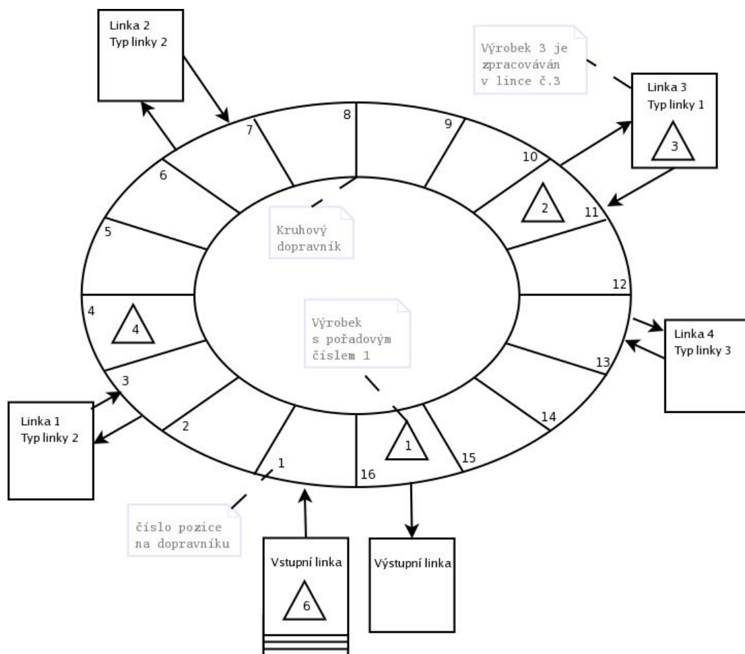
Obrázek 3: Kruhový dopravník
