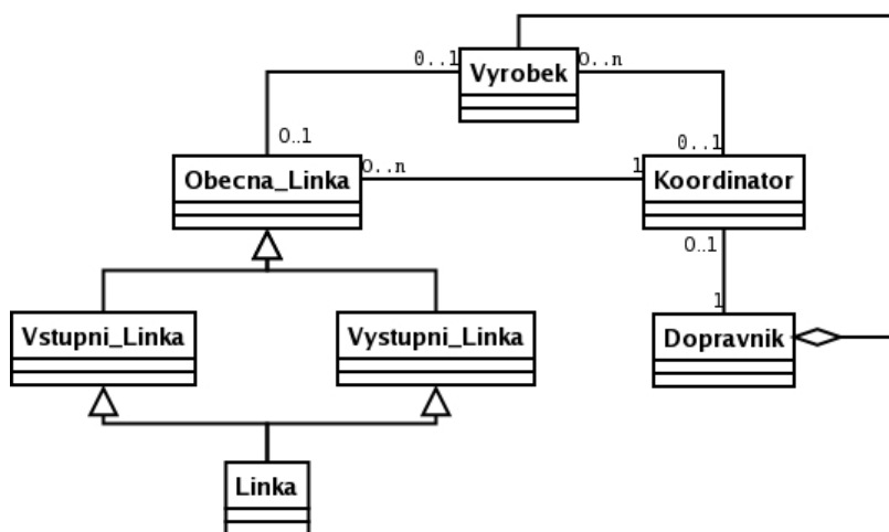
Obrázek 4: Objektový návrh
