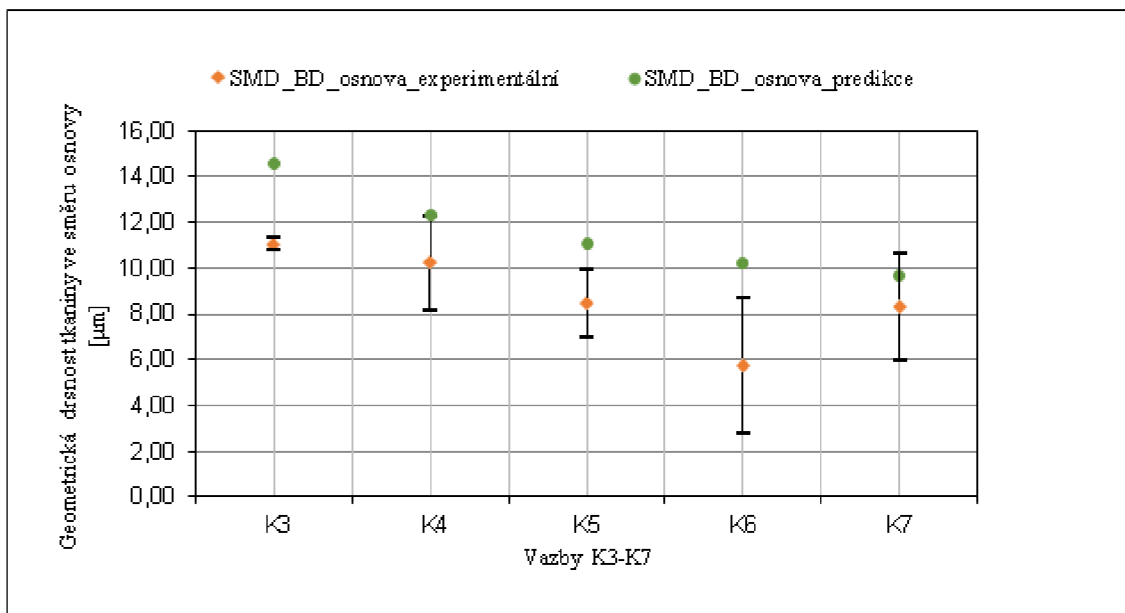
Obr. 49 Graf porovnání experimentálních a predikčních hodnot geometrické drsnosti tkaniny ve směru osnovy u rotorové příže (BD) [vlastní zdroj]
