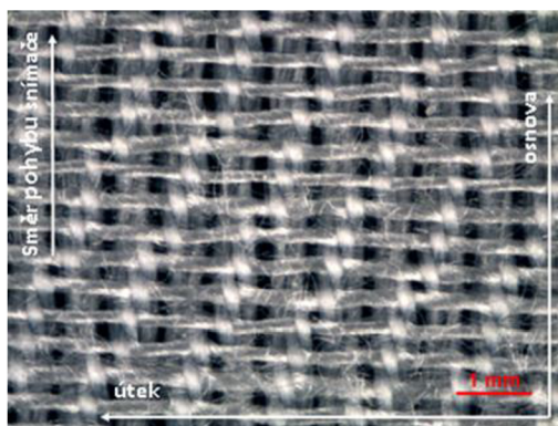
Obr. 45 Znáznornění směru snímání, SMD, tkanina PM K7 ve směru osnovy [vlastní zdroj]
