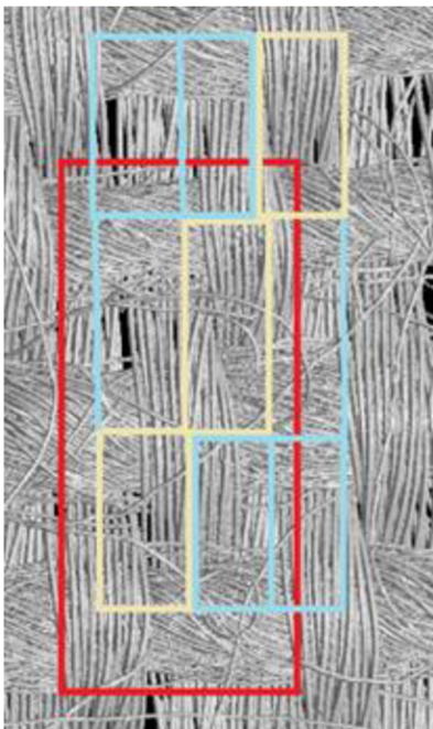
Obr. 29 Tkanina z tryskové přize (AJ) střída kepru K3-K5 [vlastní zdroj]
