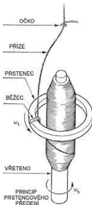
Obr. 5 Princip prstencového předení [6]
