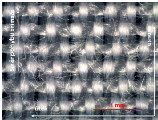
Obr. 39 Znáznornění směru snímání, SMD, tkanina PM K3 ve směru osnovy [vlastní zdroj]
