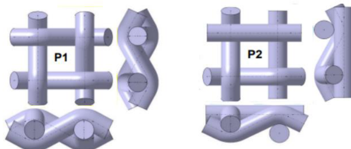
Obr. 21 Prostorové zobrazení strukturálních buněk provázání P1-P2 [45]
