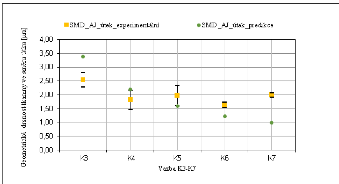
Obr. 51 Graf porovnání experimentálních a predikčních hodnot geometrické drsnosti tkaniny ve směru útku u tryskové přize (AJ) [vlastní zdroj]
