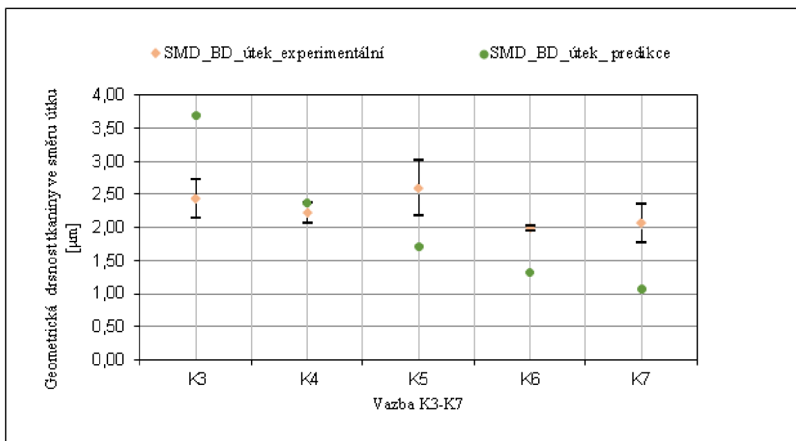
Obr. 52 Graf porovnání experimentálních a predikčních hodnot geometrické drsnosti tkaniny ve směru útku u rotorové přize (BD) [vlastní zdroj]
