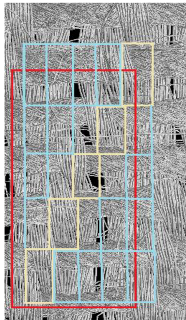
Obr. 29 Tkanina z tryskové přize (AJ) střída kepru K3-K5 [vlastní zdroj]
