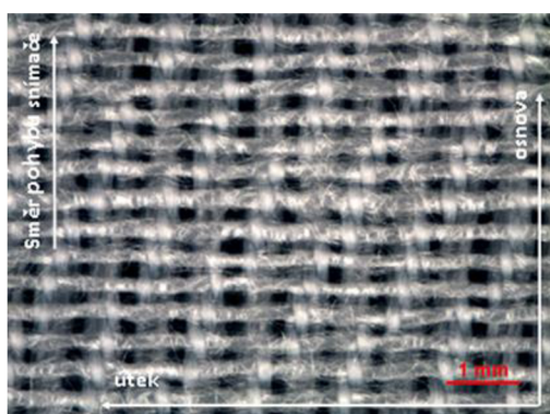
Obr. 44 Znáznornění směru snímání, SMD, tkanina BD K7 ve směru osnovy [vlastní zdroj]
