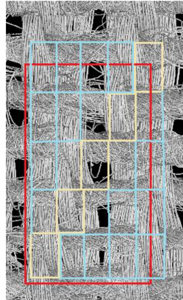
Obr. 31 Tkanina z rotorové příže (BD) střída kepru K3-K5 [vlastní zdroj]
