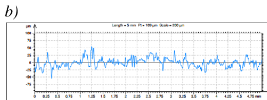
Obr. 55 Snímek plochy tkaniny BDK3 (TalyMap), rotorové příze
