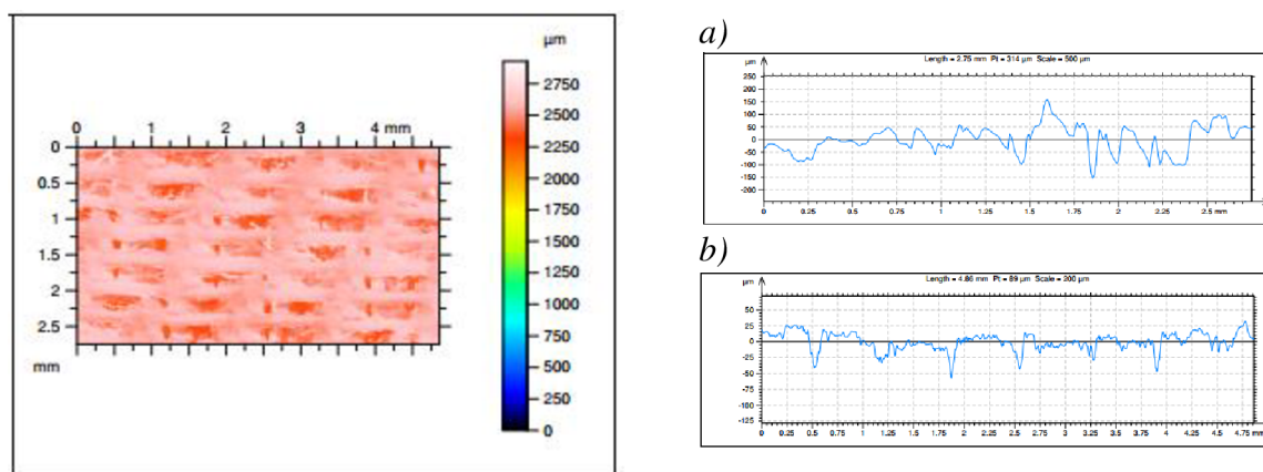
Obr. 59 Snímek plochy tkaniny PMK7 (TalyMap), prstencové mykané příže
