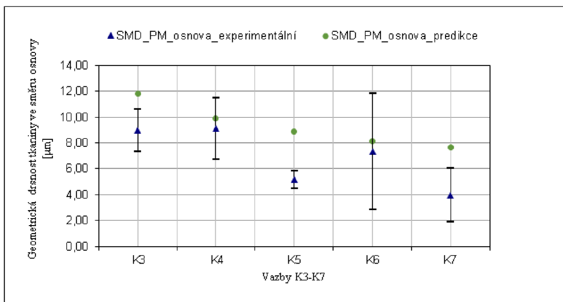
Obr. 50 Graf porovnání experimentálních a predikčních hodnot geometrické drsnosti tkaniny ve směru osnovy u prstencové mykané příže (PM) [vlastní zdroj]
