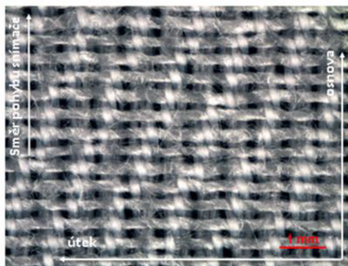
Obr. 43 Znáznornění směru snímání, SMD, tkanina AJ K7 ve směru osnovy [vlastní zdroj]
