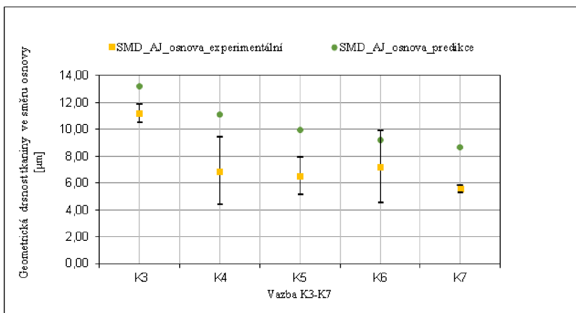
Obr. 48 Graf porovnání experimentálních a predikčních hodnot geometrické drsnosti tkaniny ve směru osnovy u tryskové přize (AJ) [vlastní zdroj]
