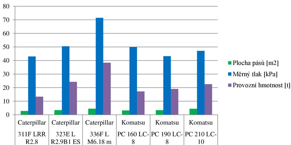
Obr. 3.11, Graf porovnání podvozků pásových rypadel [29], [30]
