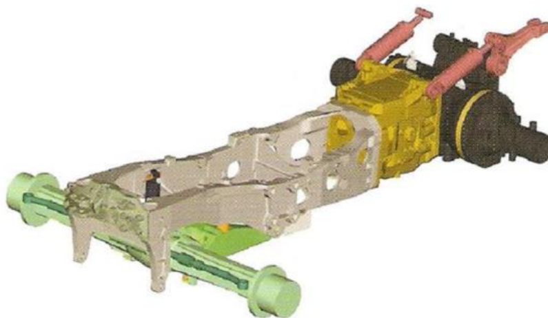
Obr. 1.7, Polorámová konstrukce traktoru [5]
