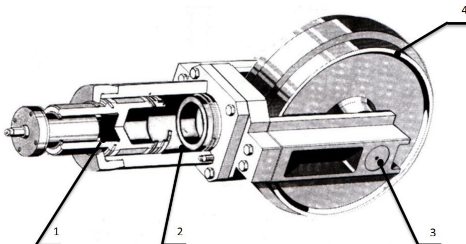
Obr. 2.7, Napínací ústrojí [13]
