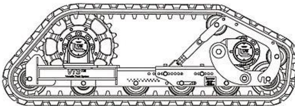
Obr. 3.1, Schématický nákres pásového podvozku VTS [14]
