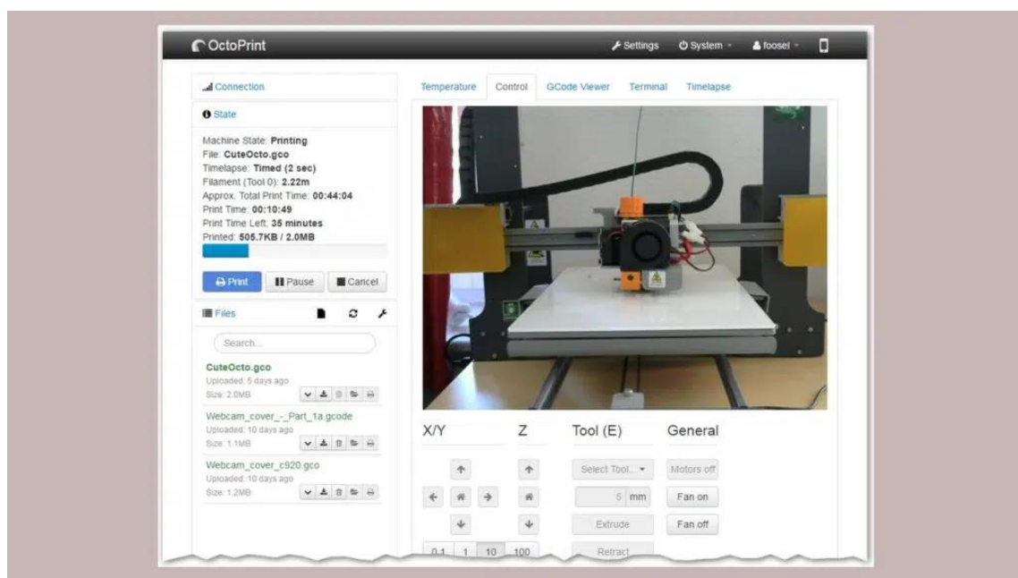
Obrázek 19 OctroPrint [57]
