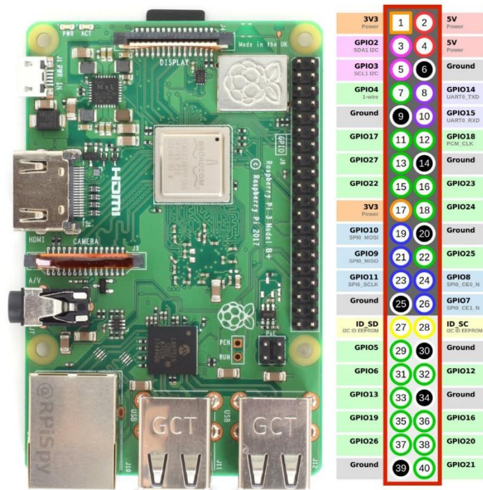
Obrázek 1 GPIO konekory [8]
