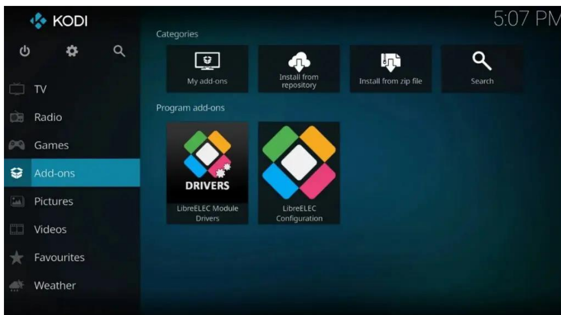
Obrázek 17 LibreELEC [53]
