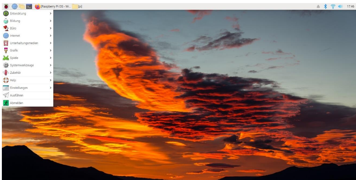
Obrázek 13 Raspbian OS [45]
