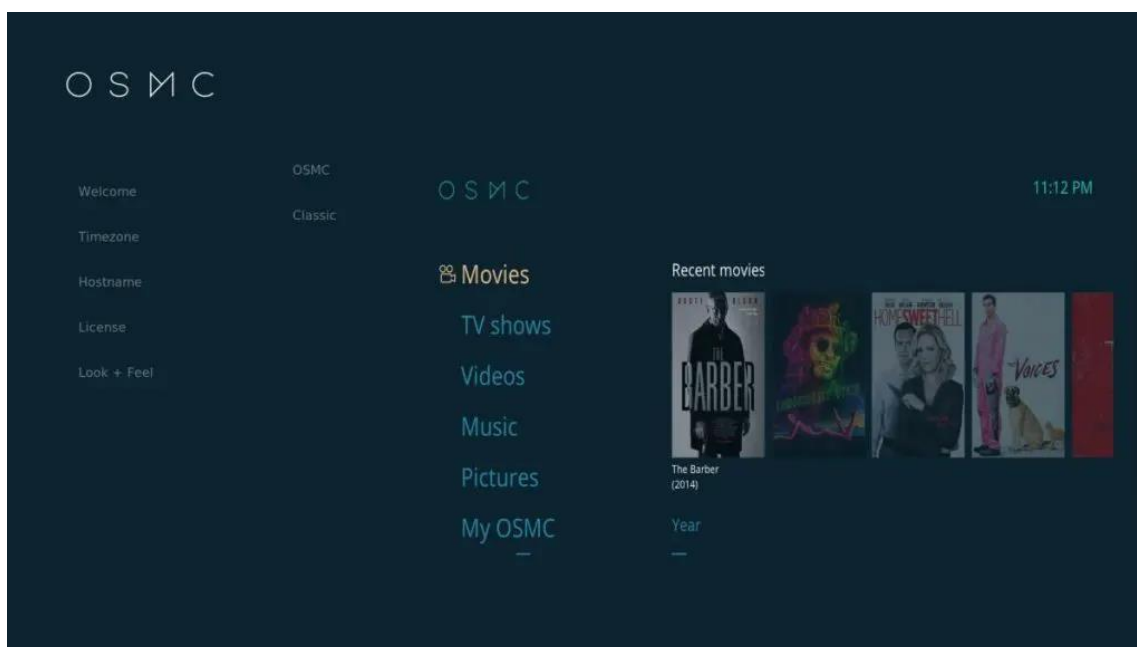
Obrázek 18 OSMC [55]
