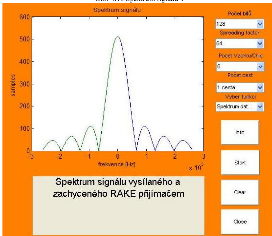
Obr. 4.11 Spektrum signálu 2
