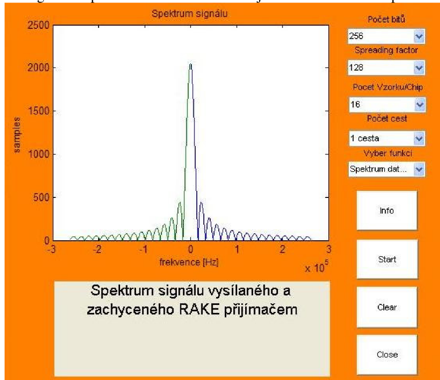
Obr. 4.10 Spektrum signálu 1
