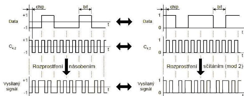
Obr. 2.1 Příklad rozprostírání datového signálu [ 1 ]
