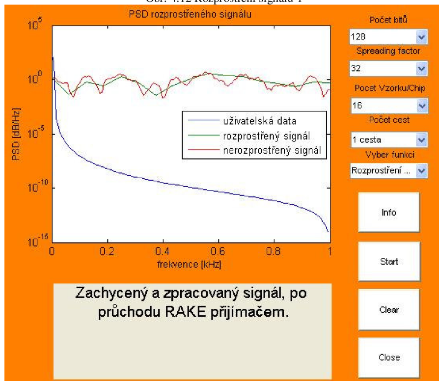
Obr. 4.13 Rozprostření signálu 2
