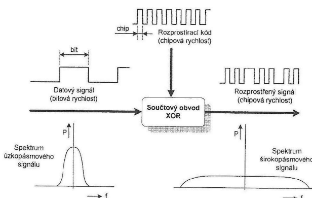
Obr. 2.3 Příklad rozptření signálu technikou DS-SS [ 1 ]
