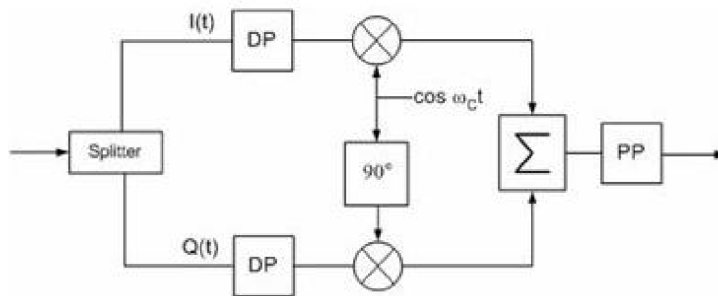
Obr. 2.8 Blokové schéma QPSK modulátoru [ 17 ]
