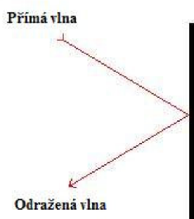
Obr. 3.3 Odraz vlny
