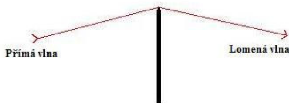
Obr. 3.4 Lom vlny
