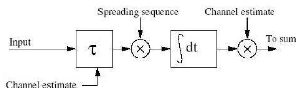
Obr. 3.1 RAKE finger [ 9 ]
