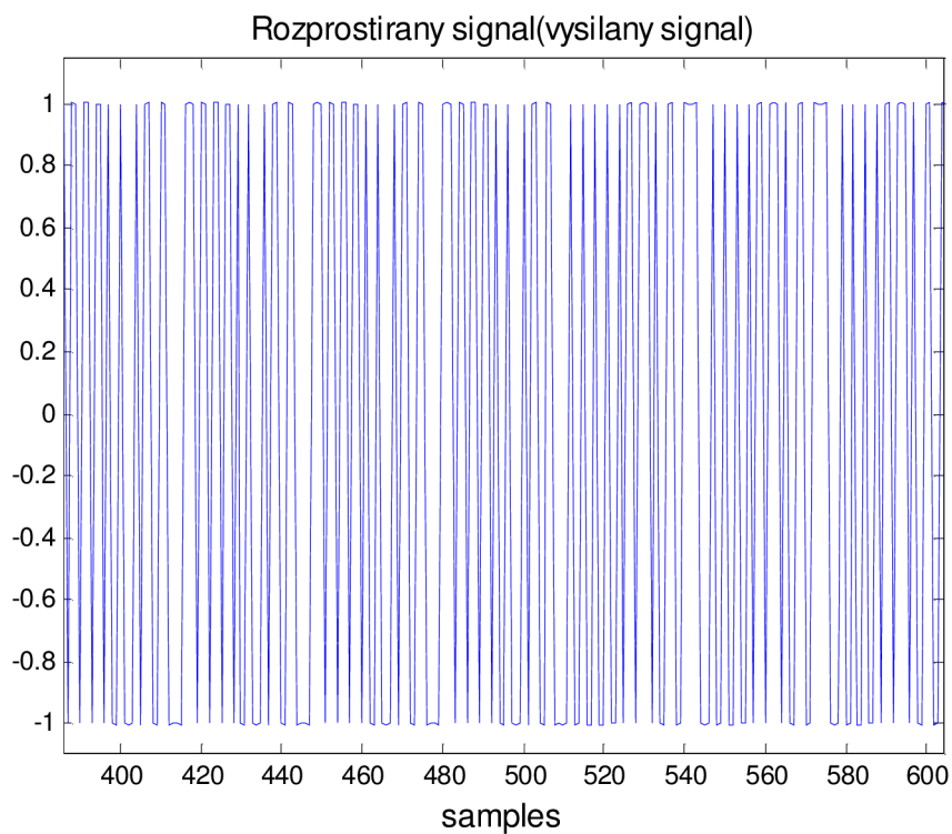
Obr. 4.6 Rozprostřaný signál
