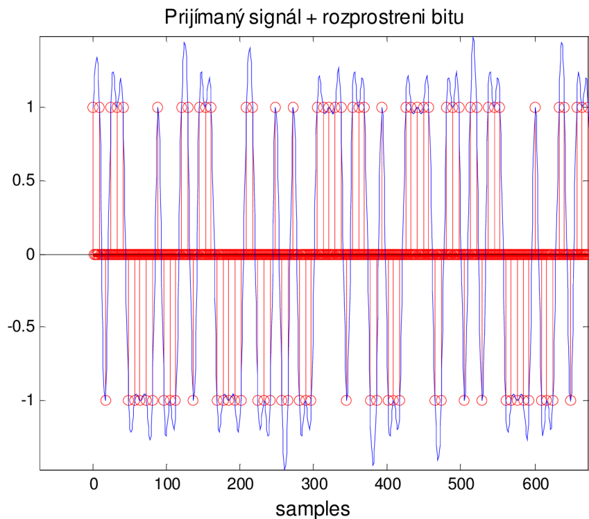
Obr. 4.3 Přijímaný signál + rozprostření bitů
