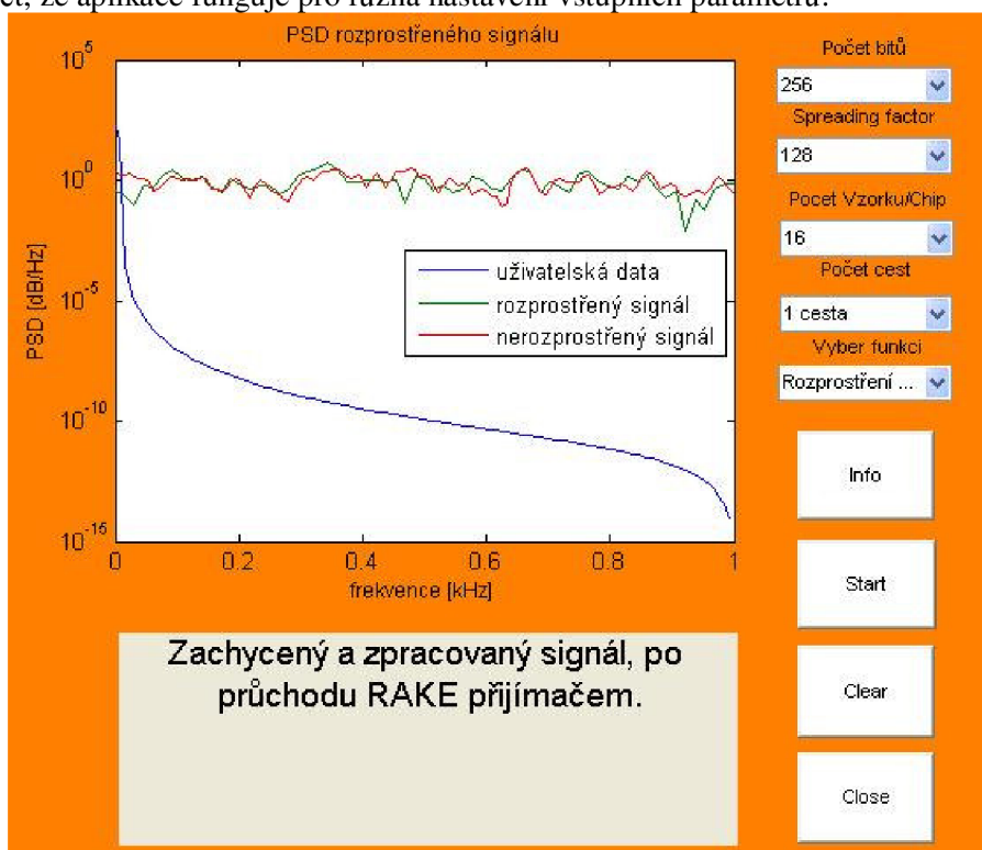
Obr. 4.12 Rozprostření signálu 1
