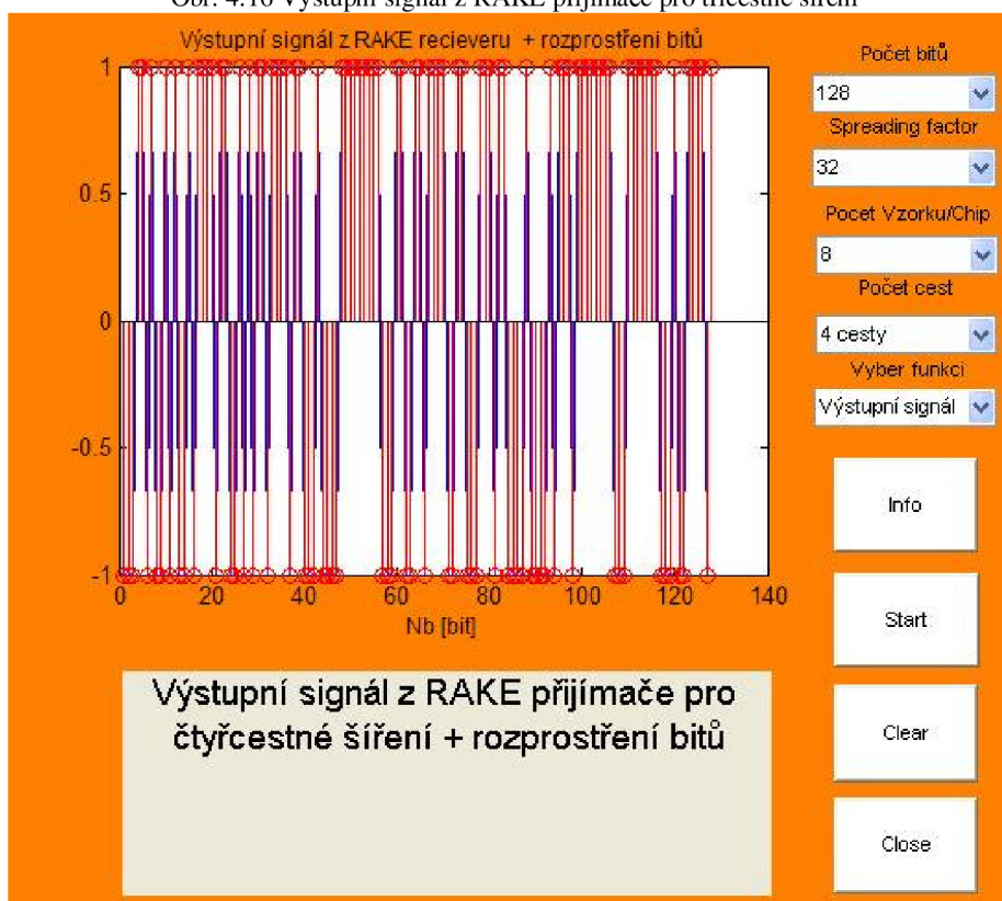
Obr. 4.17 Výstupní signál z RAKE přijímače pro čtyřcestné šíření
