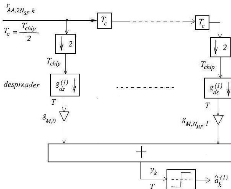
Obr. 3.8 RAKE přijímač s derozprostíračem [ 2 ]
