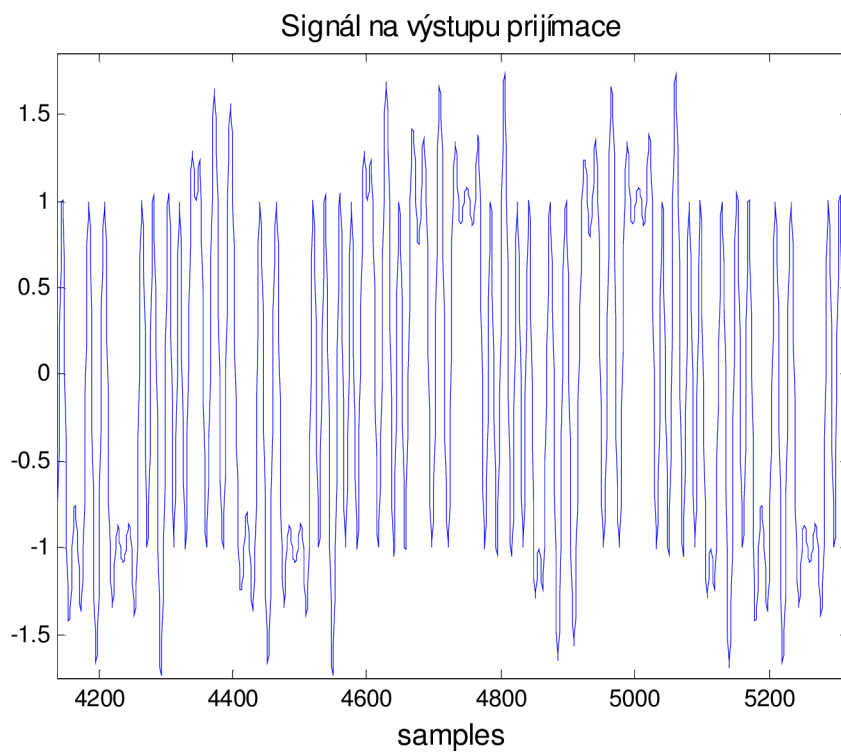
Obr. 4.5 Signál na výstupu přijímače
