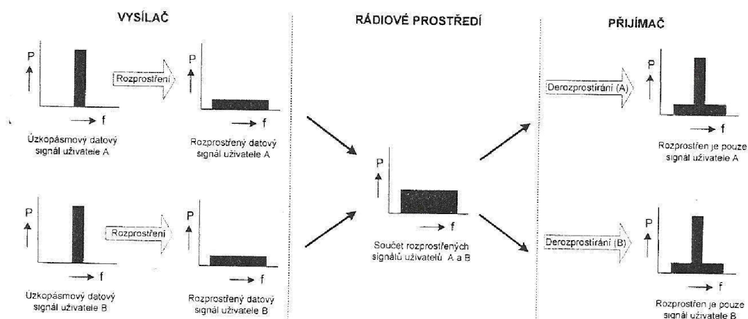
Obr. 3.9 Příklad přenosu signálu v CDMA [ 1 ]
