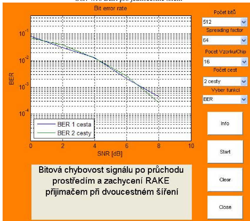
Obr. 4.19 BER pro dvoucestné šíření
