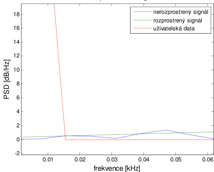
Obr. 4.2 PSD rozprostřeného signálu
