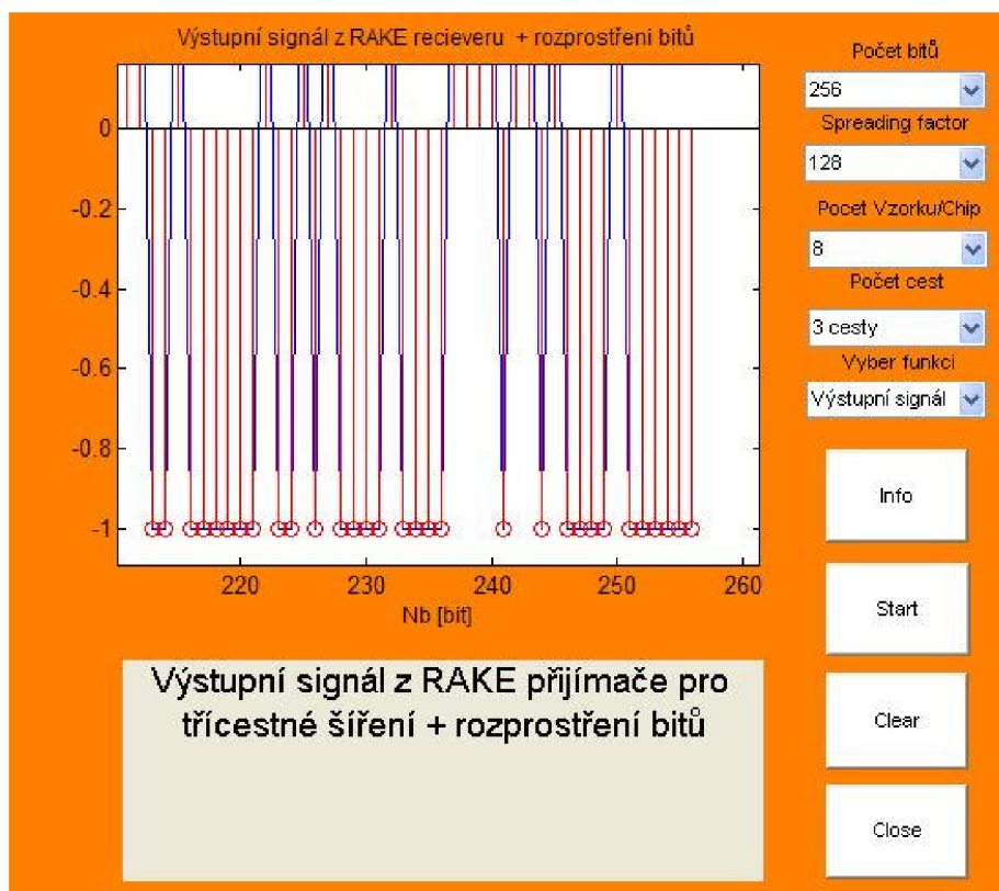
Obr. 4.16 Výstupní signál z RAKE přijímače pro třicestné šíření
