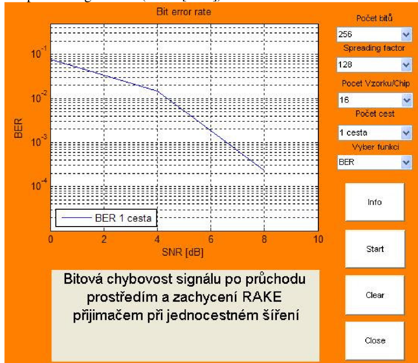
Obr. 4.18 BER pro jednocestné šíření
