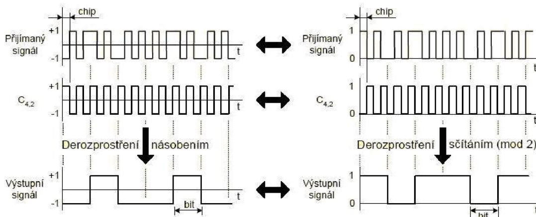
Obr. 2.5 Příklad derozprostření datového signálu [ 1 ]
