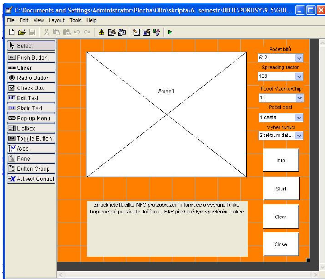
Obr. 4.8 Rozložení komponent aplikace
