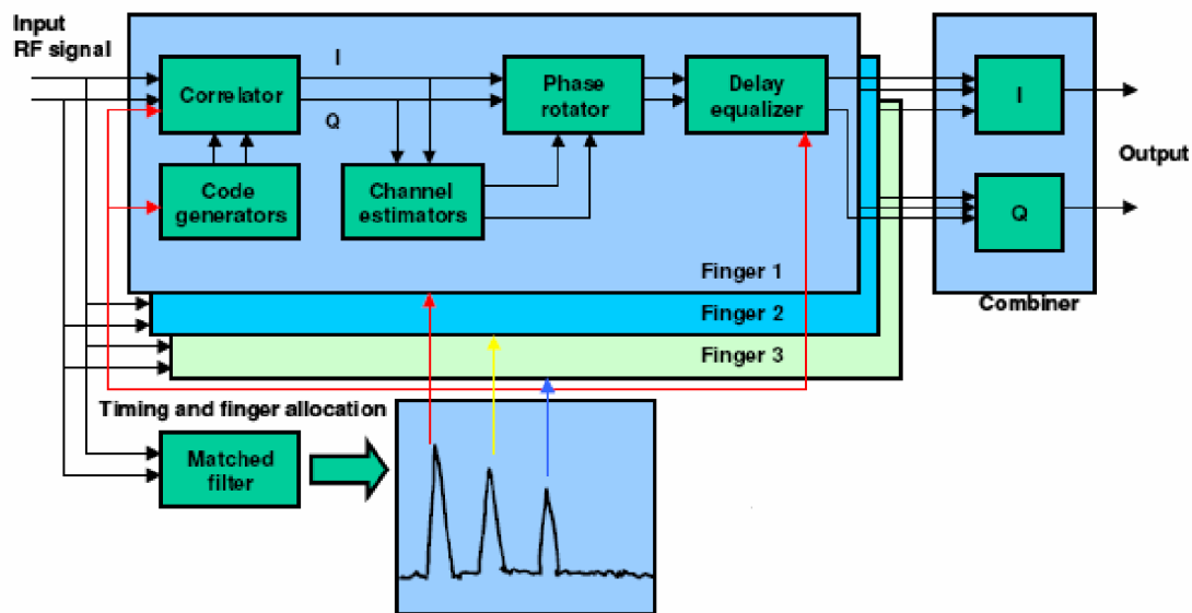
Obr. 3.6 Blokové schéma RAKE přijímače [ 5 ]
