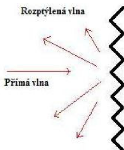
Obr. 3.5 Rozptyl vlny
