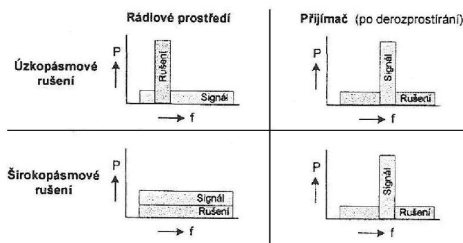
Obr. 2.4 Vliv úzkopásmového a širokopásmového rušení [ 1 ]
