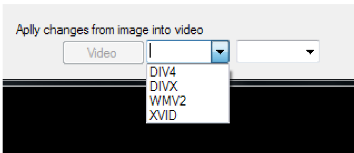
Obr. 2.14: Ponuka kodekov
