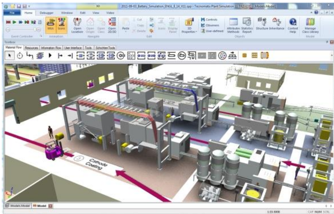
Obrázek 15 – Prostředí programu Tecnomatix Plant Simulation [16]
