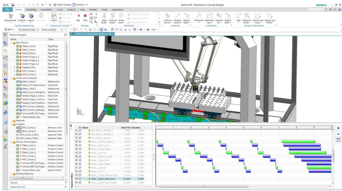
Obrázek 13 – Simulace modelu pomocí NX Process Simulate [35]
