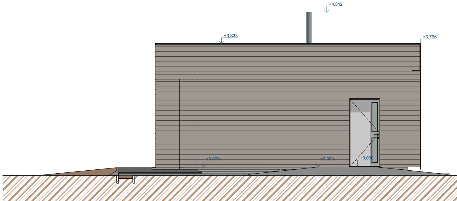
Pohled východní
