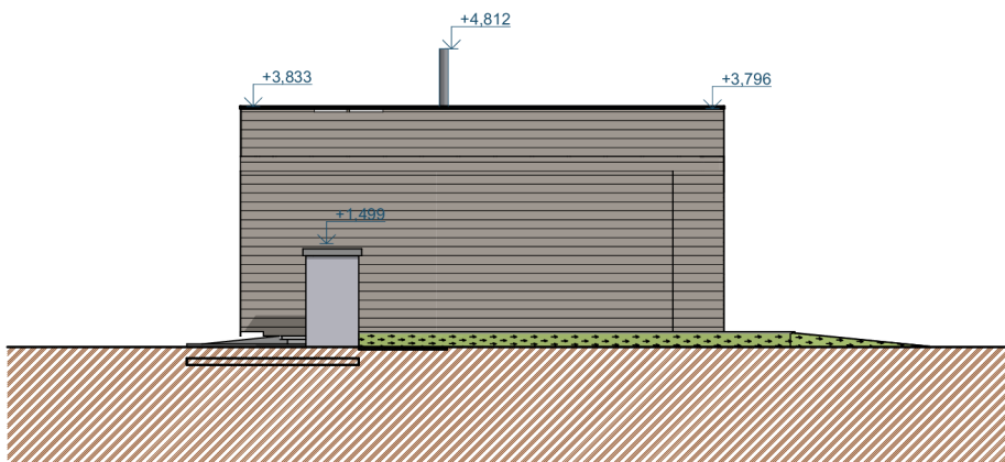
Pohled východní
