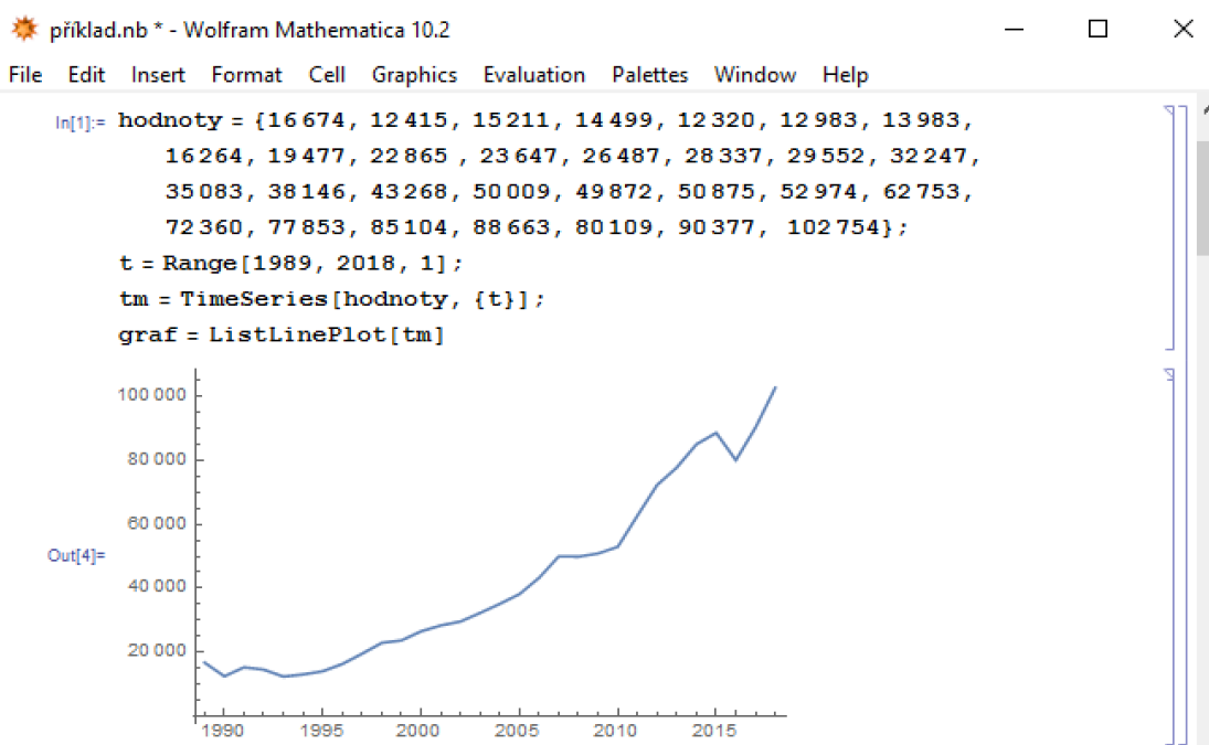
Obrázek 17 Vývoj hodnot časové řady
