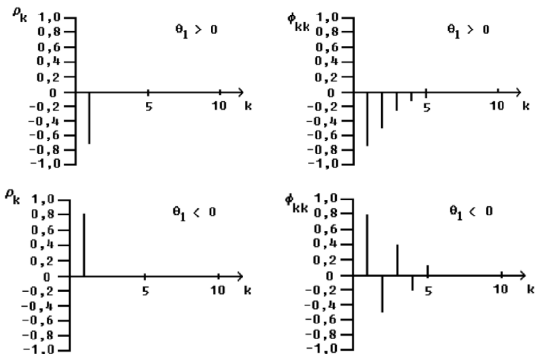
Obrázek 6 ACF a PACF modelu MA(1)
